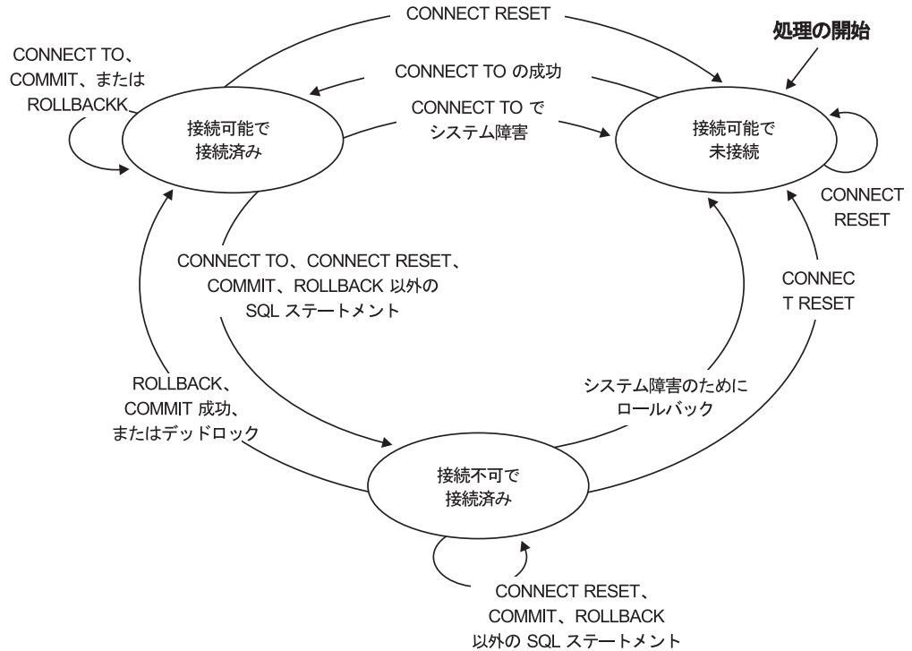
図 10. 暗黙的接続が可能でない場合の接続状態遷移
