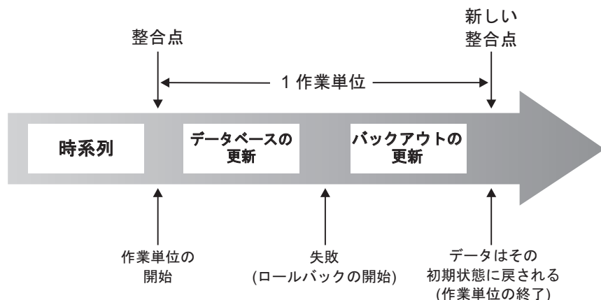
図 5. ROLLBACK ステートメントの作業単位
