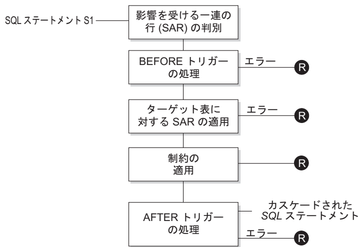
図 18. 関連するトリガーと制約を伴うステートメントの処理
