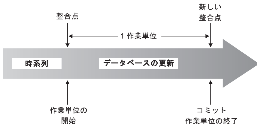
図4. COMMIT ステートメントの作業単位
