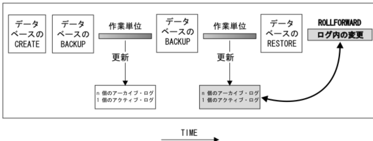
図 19. データベースのロールフォワード・リカバリ：長時間実行しているトランザクションの場合には、複数のアクティブ・ログが生じる可能性があります。
