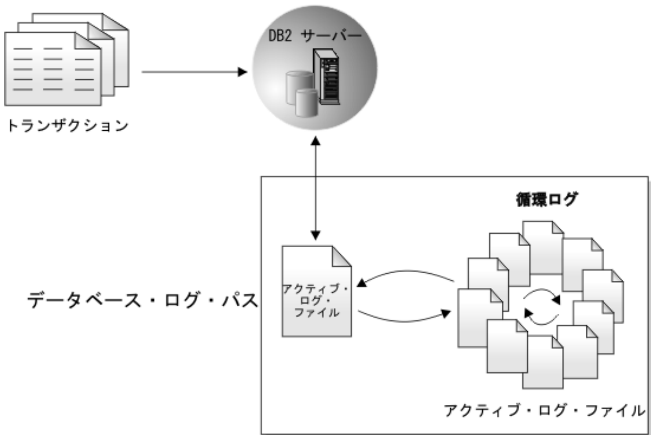
図1. 循環ロギング
