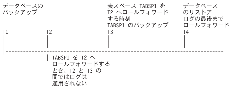
図 24. 表スペースのバックアップ要件
