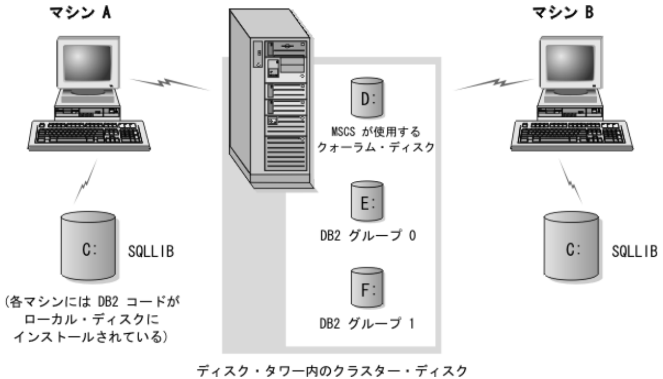
図 3. Failover Clustering の構成の例
