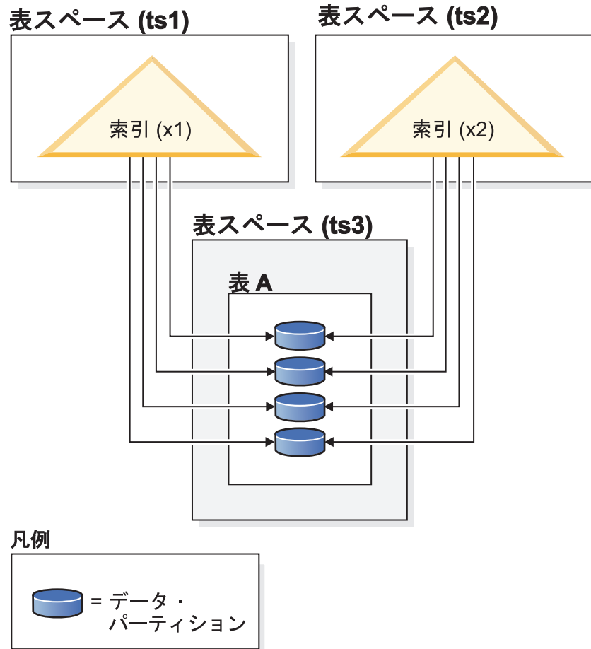
図 50. パーティション表上の非パーティション化索引
