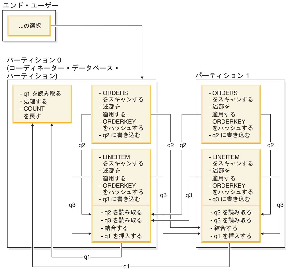
図 58. 内部表および外部表の指示結合の例
