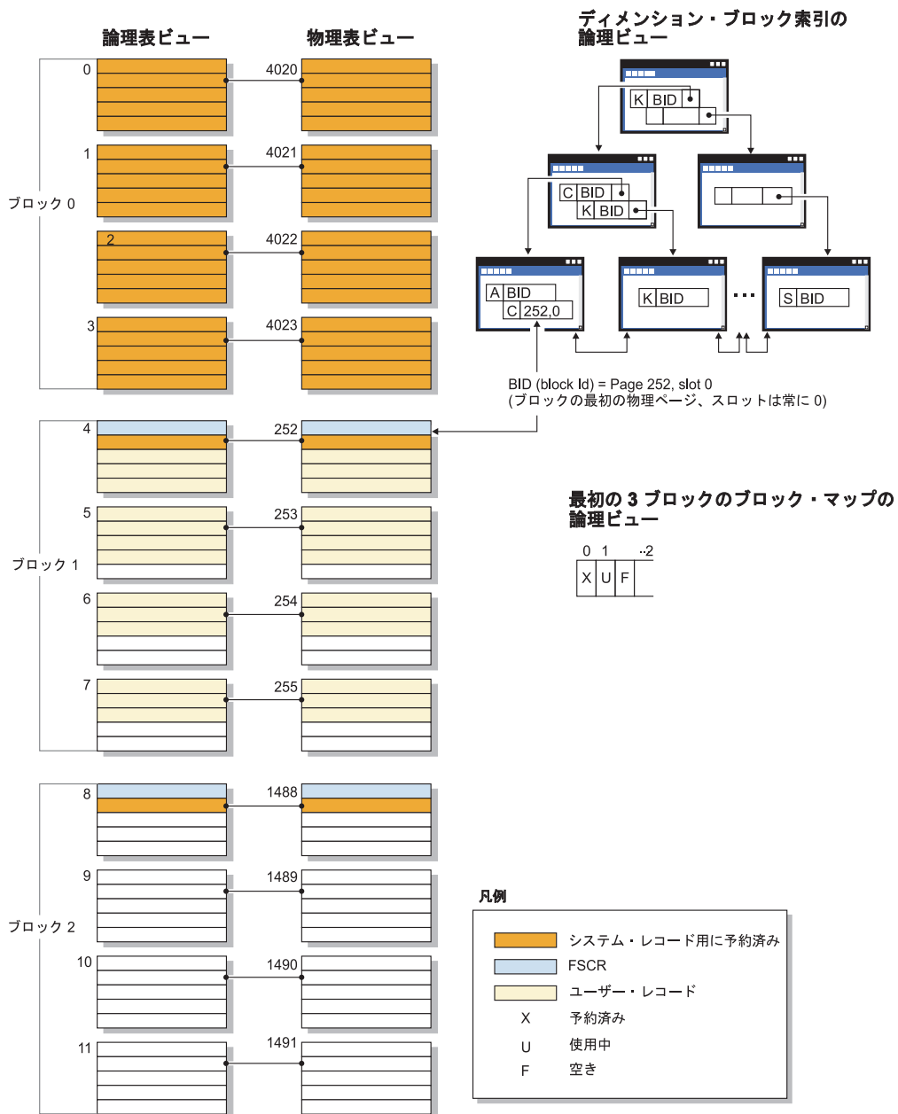
図 54. MDC 表の論理表、レコード、および索引構造
