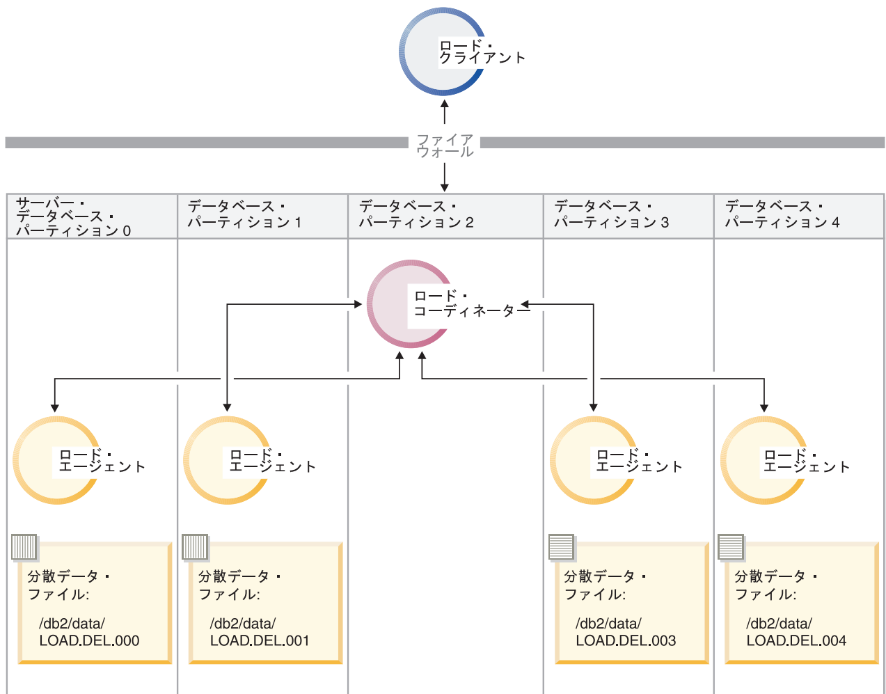
図 44. 特定の表が定義されているすべてのデータベース・パーティションへのデータのロード。： この図では、前のコマンドが発行された結果の動作を説明します。分散データは、TABLE1 が定義されているすべてのデータベース・パーティションにロードされます。
