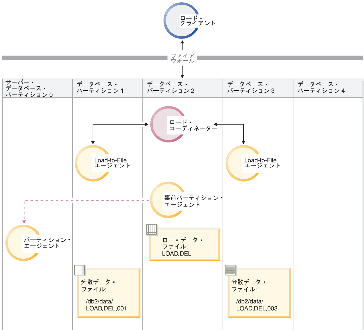
図 43. 1 つのパーティション化エージェントを使用したデータベース・パーティション 1 および 3 へのデータのロード。： この図では、前のコマンドが発行された結果の動作を説明します。データは、データベース・パーティション 0 で実行する 1 パーティション化エージェントを使用して、データベース・パーティション 1 および 3 にロードされます。
