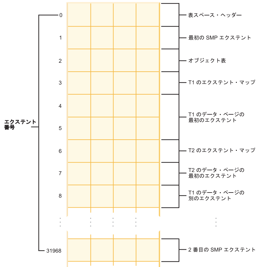
図9. 論理表スペース・アドレス・マップ
