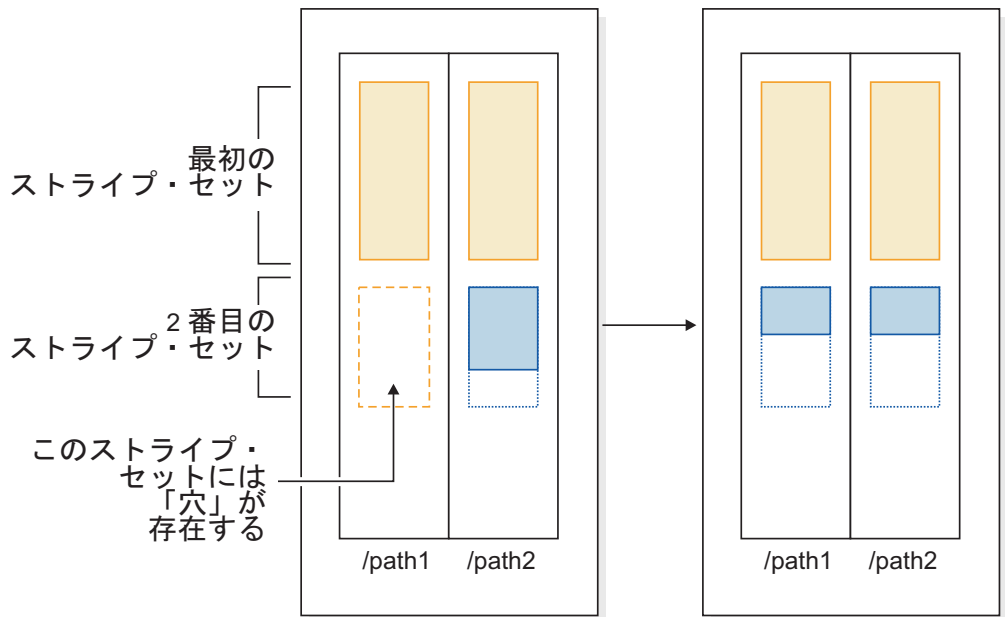
図 28. ギャップを埋めるための自動ストレージ表スペースのリバランス
