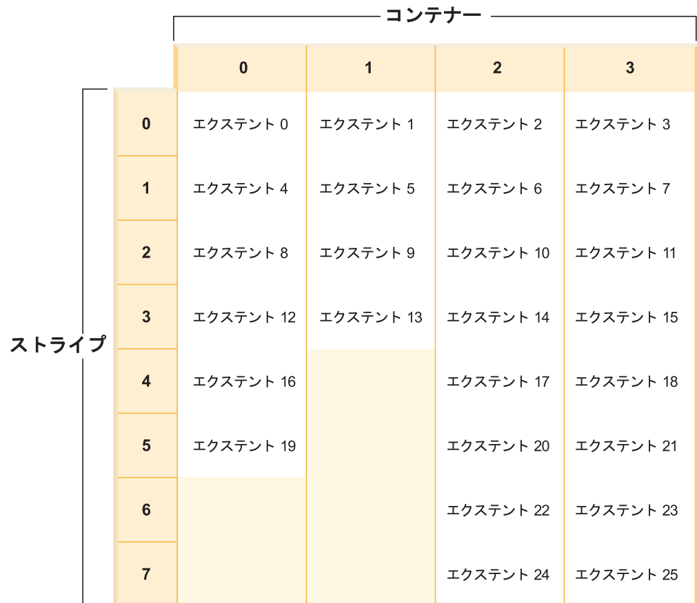
図 20. 4 つのコンテナ、26 のエクステントが含まれる表スペース
