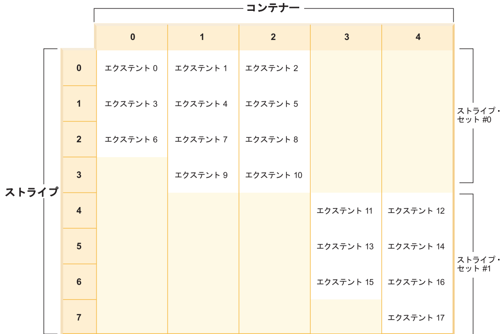
図 26. 2 つのストライプ・セットを含む表スペース
