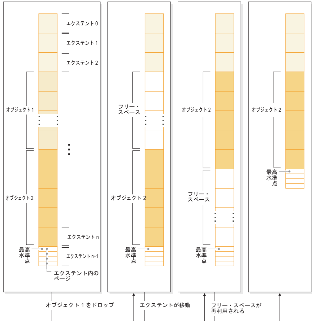
図 17. 再利用可能ストレージ機能の仕組み：表スペースで再利用可能ストレージが使用可能な場合、使用中のエクステントを移動して、表スペース内の低い位置にある未使用のエクステントを占有できます。
