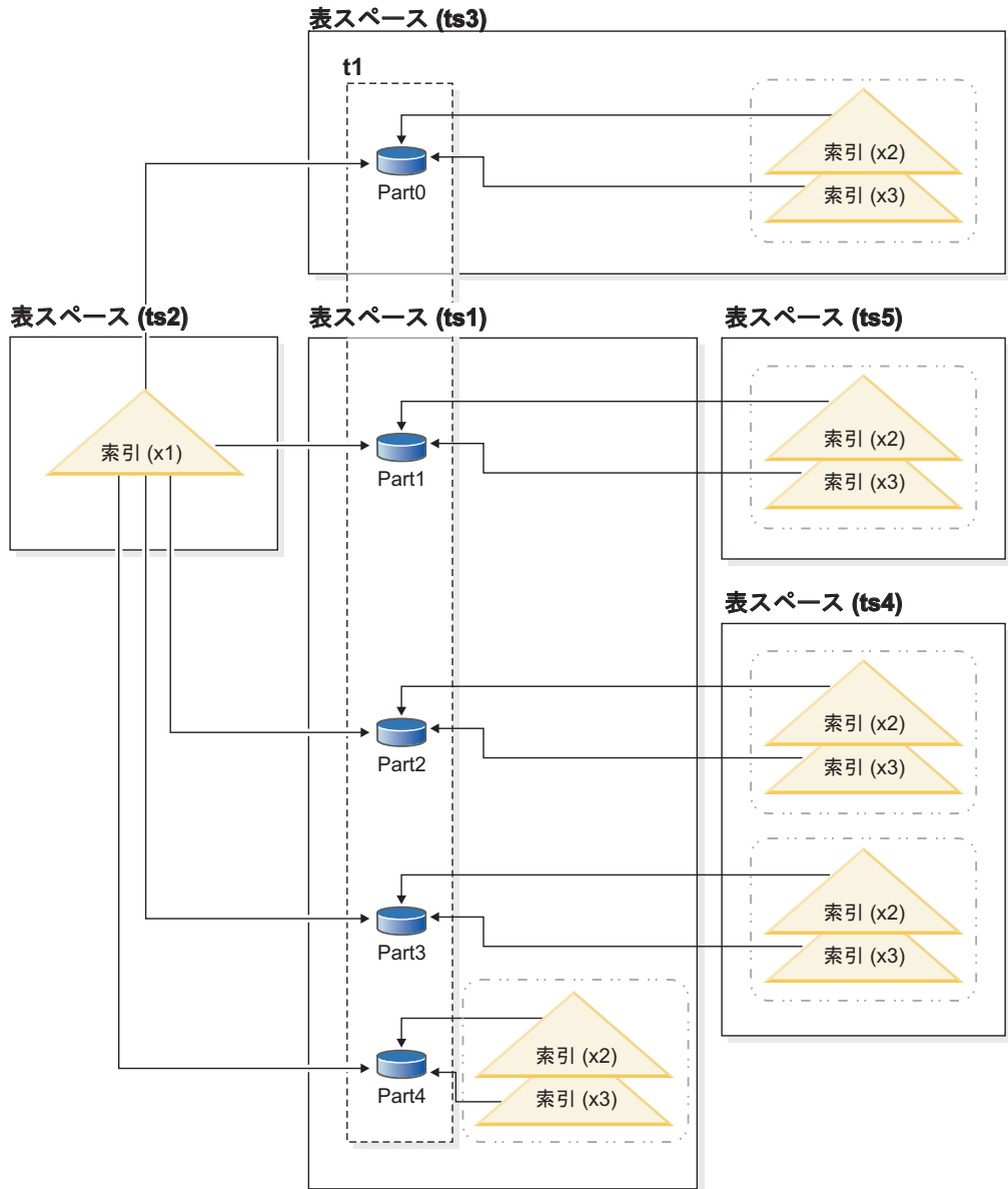
図 44. パーティション表の非パーティション索引とパーティション索引の組み合わせ
