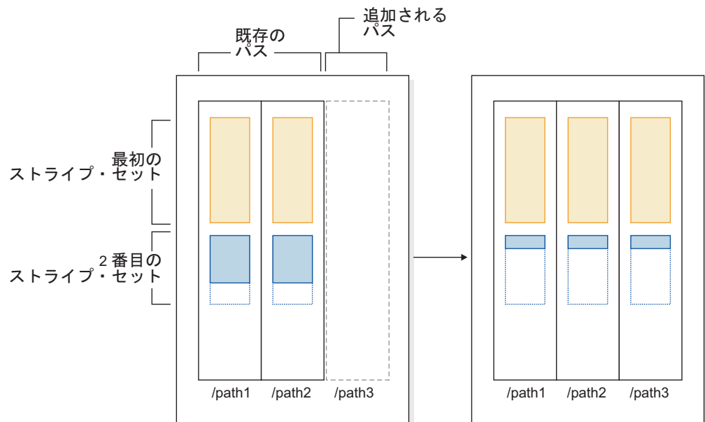
図 15. 新しいストレージを追加して、表スペースをリバランスした場合の結果
