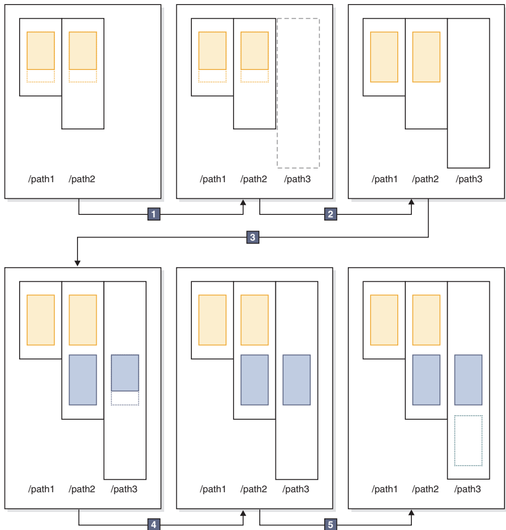
図 14. 必要に応じて、自動ストレージがコンテナを追加する方法
