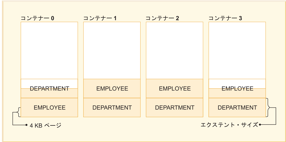
図 8. 表スペースの中のコンテナとエクステンツ
