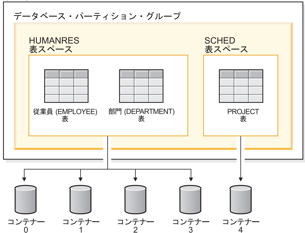
図7. データベース内の表スペースと表
