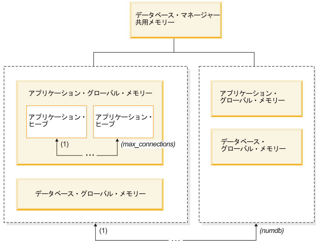
図1. データベース・マネージャーによって割り振られるメモリーのタイプ
