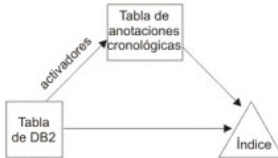
Figura 2. Proceso de actualización incremental con activadores
