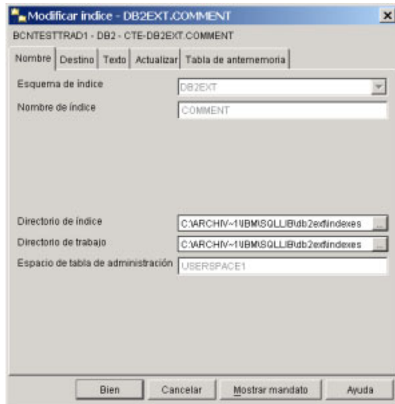
Figura 20. Recuadro de diálogo Modificar índice: pestaña Nombre
