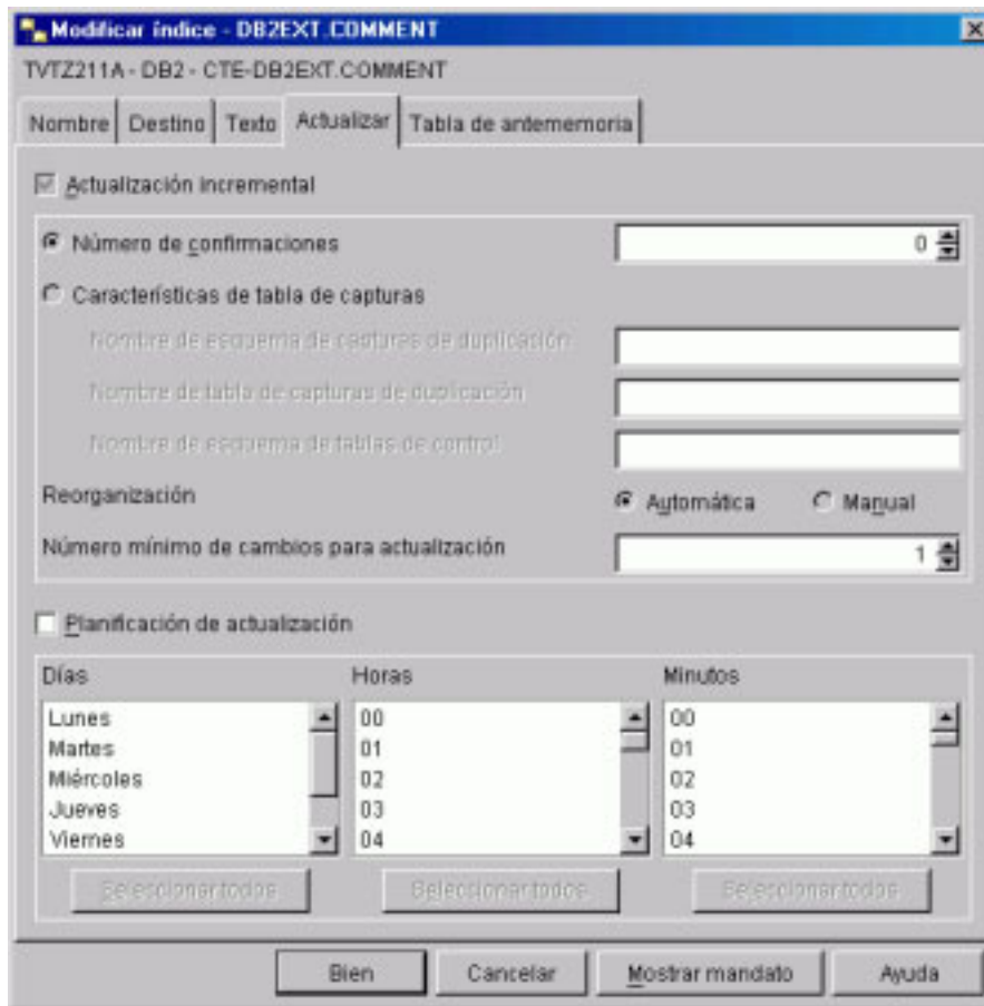
Figura 21. Recuadro de diálogo Modificar índice: pestaña Actualizar
