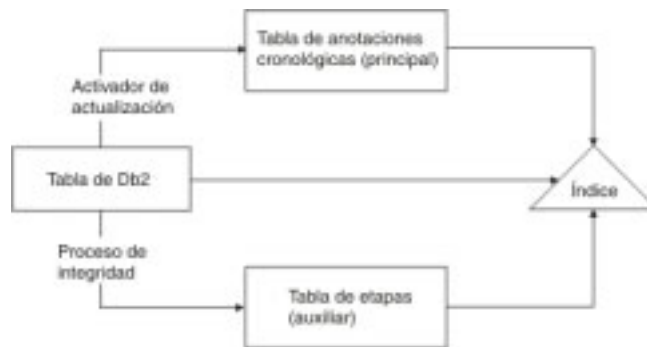
Figura 3. Actualizaciones incrementales con activadores y proceso de integridad
