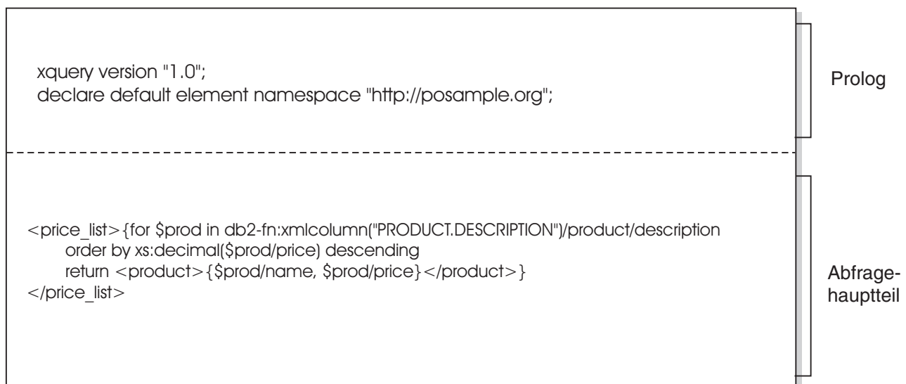
Abbildung 4. Struktur einer typischen XQuery-Abfrage
