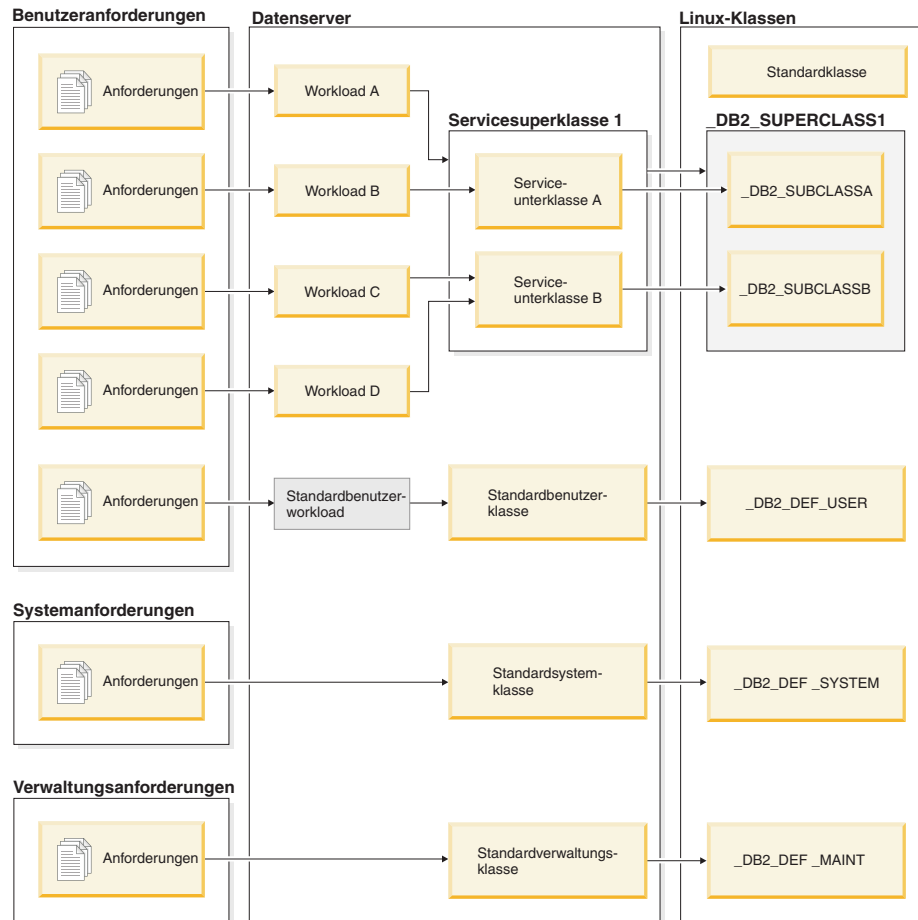
Abbildung 31. Integration von DB2-Workload-Manager und Linux-Workload-Management
