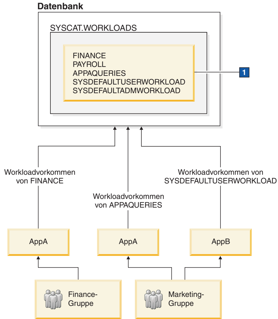
Abbildung 6. Beispiel einer Workloadzuordnung
