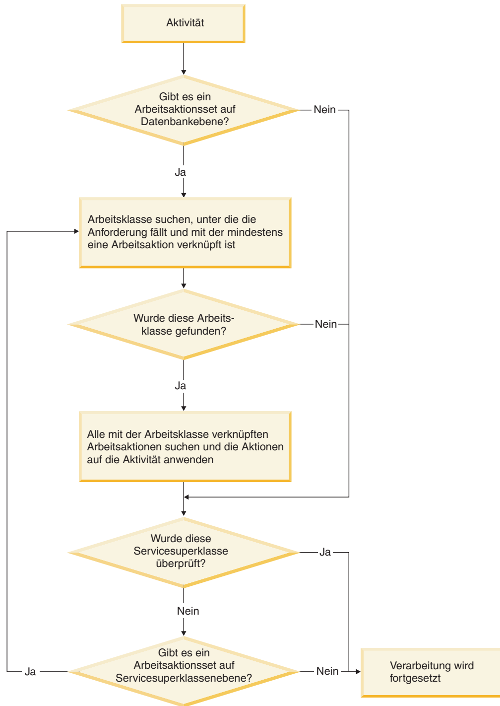
Abbildung 20. Anwenden einer Arbeitsaktion auf eine Aktivität
