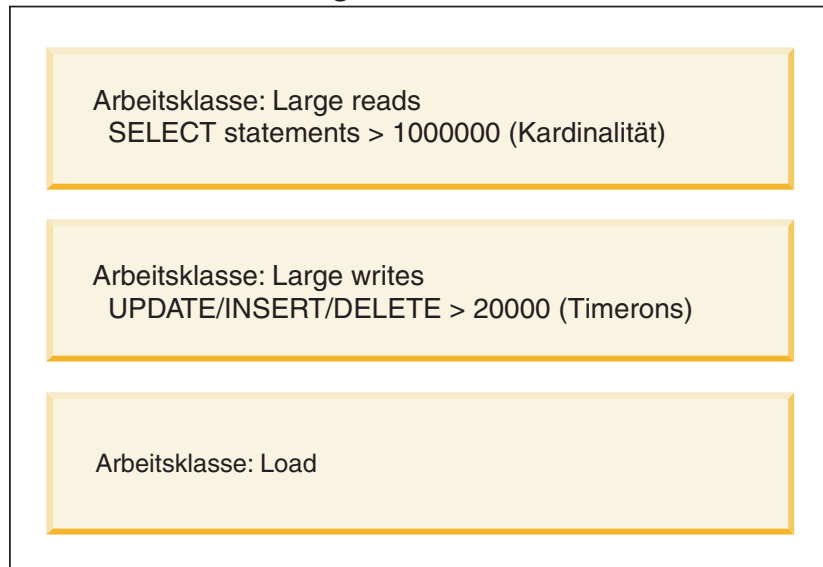
Abbildung 9. Beispiel von Arbeitsklassen in einem Arbeitsklassenset
