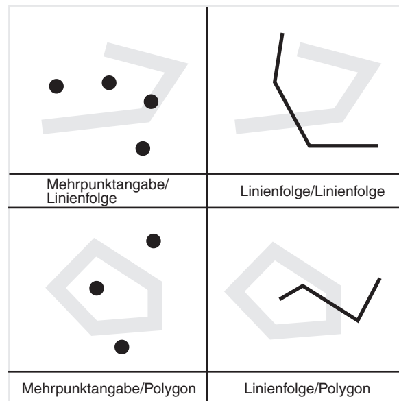
Abbildung 46. ST_Crosses
