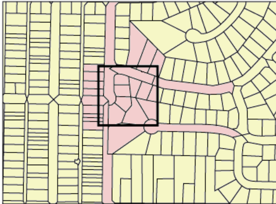
Abbildung 13. Benachbarte Landparzellen
