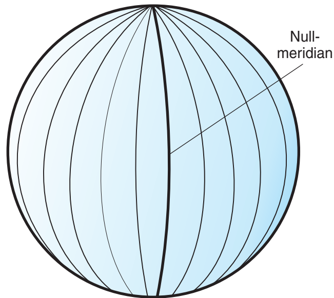
Abbildung 8. Längengradlinien
