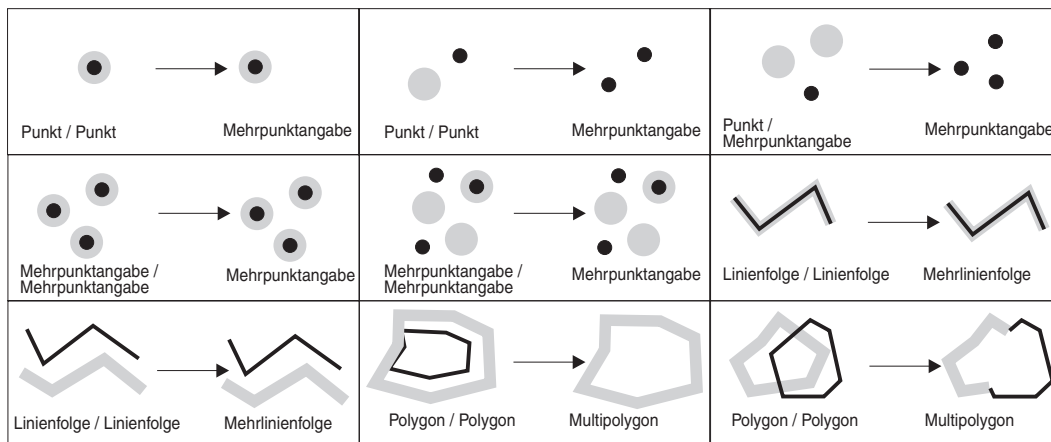
Abbildung 55. ST_Union
