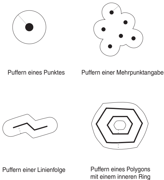
Abbildung 51. ST_Buffer
