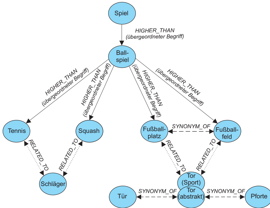
Abbildung 29. Beispiel für die Struktur eines Thesaurus
