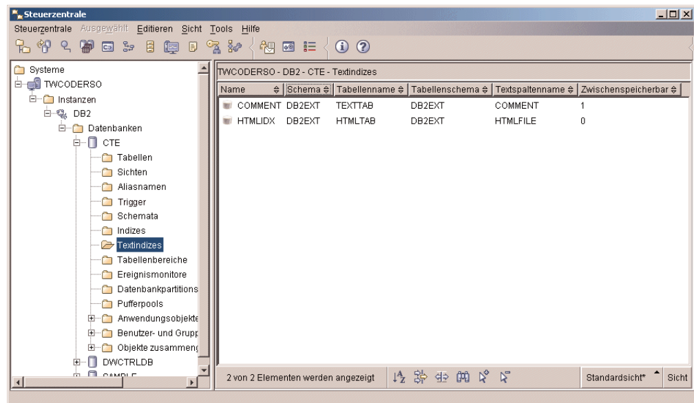
Abbildung 7. DB2-Steuerzentrale
