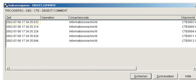
Abbildung 25. Dialog 'Indexereignisse'
