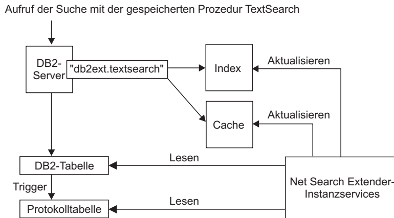
Abbildung 5. Verwenden einer Suche mit gespeicherten Prozeduren
