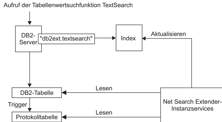
Abbildung 6. Ausführung von Suchoperationen mit einer SQL-Tabellenwertfunktion
