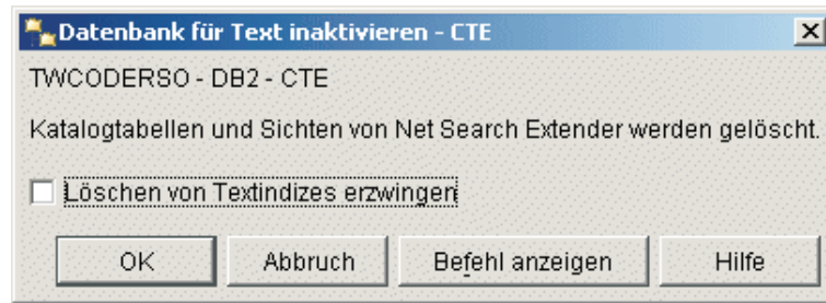
Abbildung 9. Dialog 'Datenbank für Text inaktivieren'
