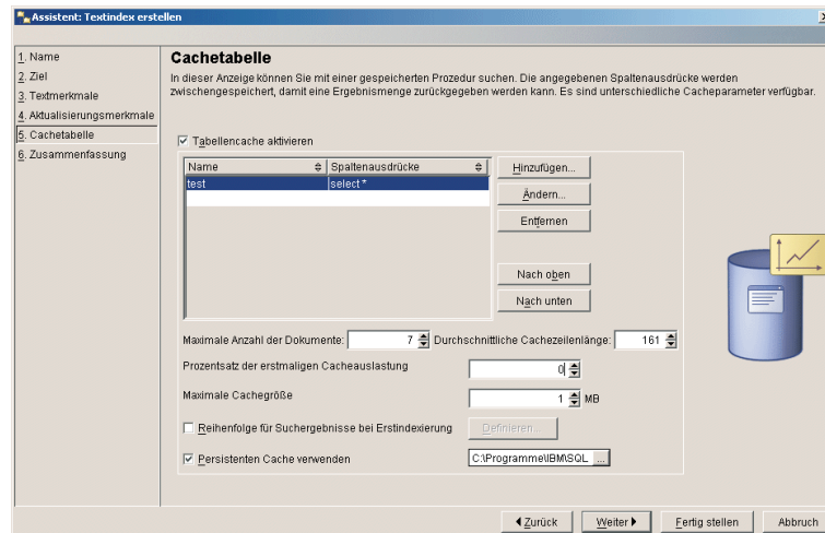
Abbildung 16. Assistent: Textindex erstellen - Anzeige 'Cachetabelle'
