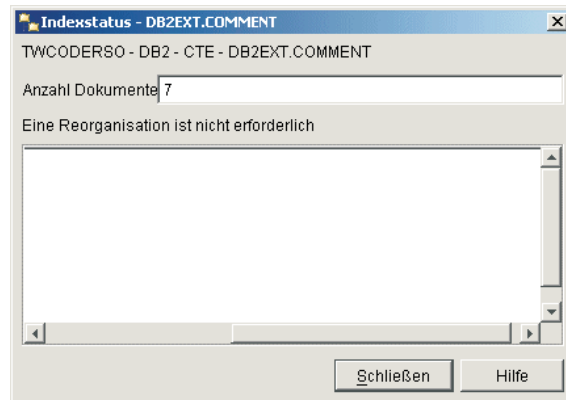
Abbildung 28. Dialog 'Indexstatus'
