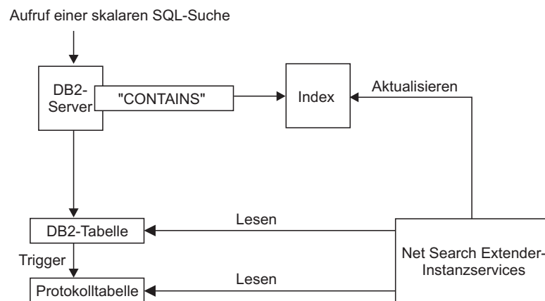
Abbildung 4. Ausführung von Suchoperationen mit einer skalaren SQL-Suchfunktion
