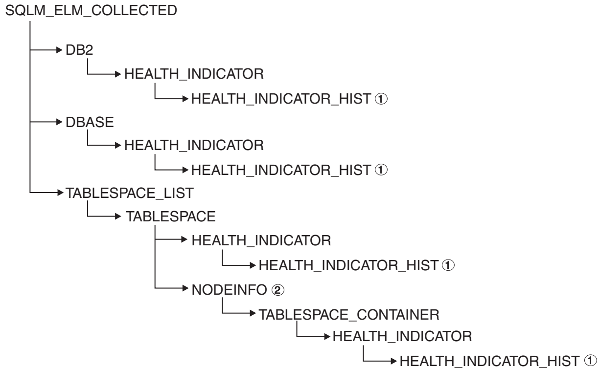
Abbildung 5. Selbstbeschreibender Datenstrom zu einer Diagnosemomentaufnahme
