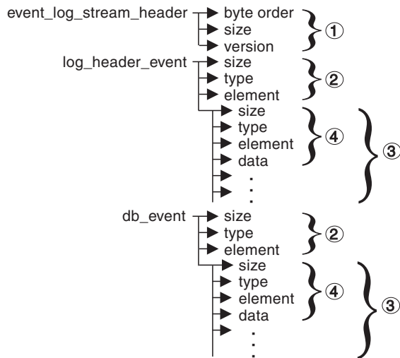
Abbildung 1. Datenstrom eines Ereignismonitors
