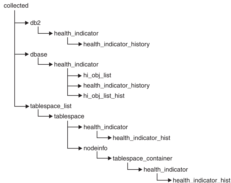
Abbildung 6. Logische Datengruppierungen einer Diagnosemomentaufnahme
