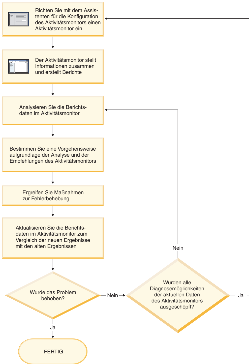
Abbildung 7. Übersicht über den Aktivitätsmonitor
