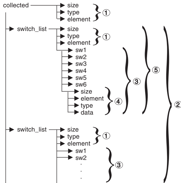
Abbildung 3. Datenstrom für Monitorschalterlisten
