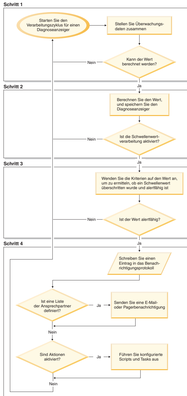
Abbildung 4. Verarbeitungszyklus für Diagnoseanzeiger
