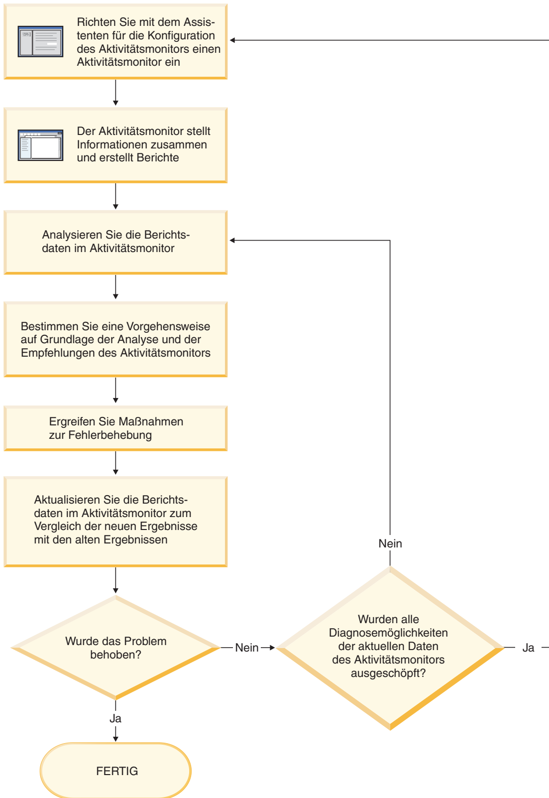
Abbildung 7. Übersicht über den Aktivitätsmonitor
