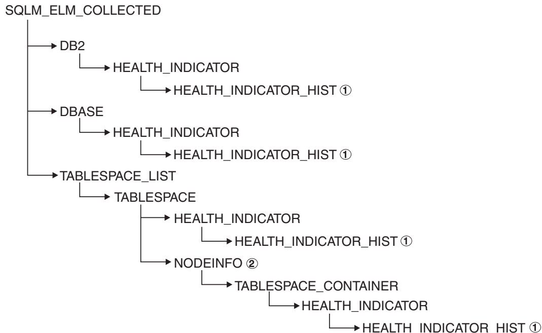
Abbildung 5. Selbstbeschreibender Datenstrom zu einer Diagnosemomentaufnahme
