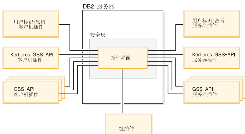
图 4. 在 DB2 服务器上部署安全插件
