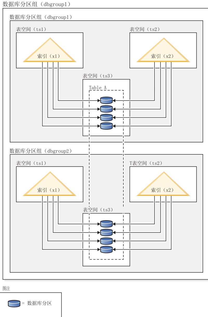
图 51. 分布式分区表的索引行为
