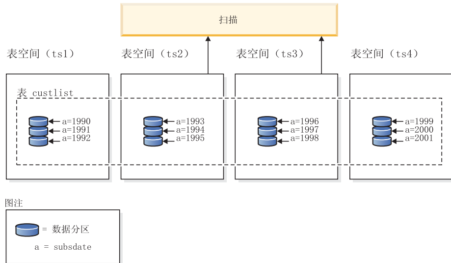
图 48. 分区表上数据分区消除所产生的性能方面的好处
