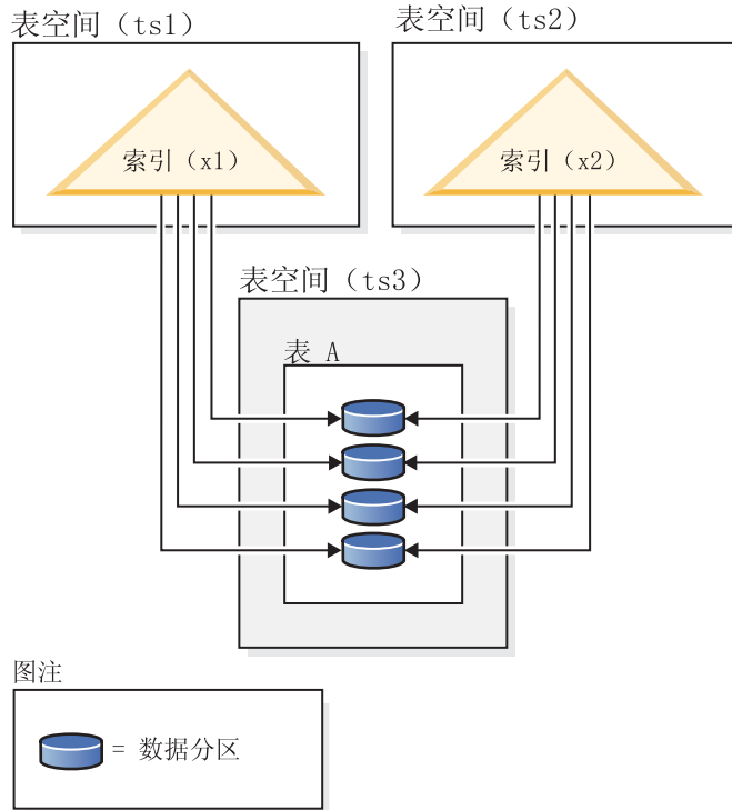
图 50. 分区表上的索引行为
