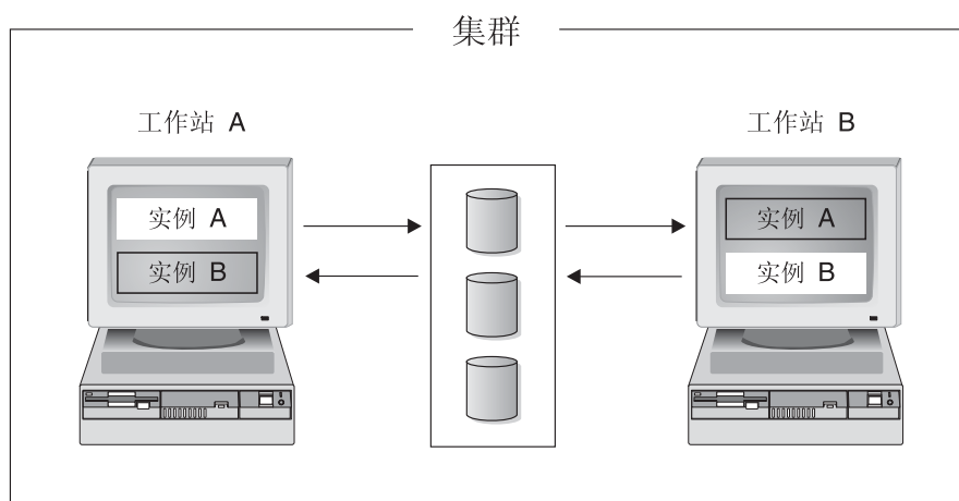
图 5. 相互接管配置
