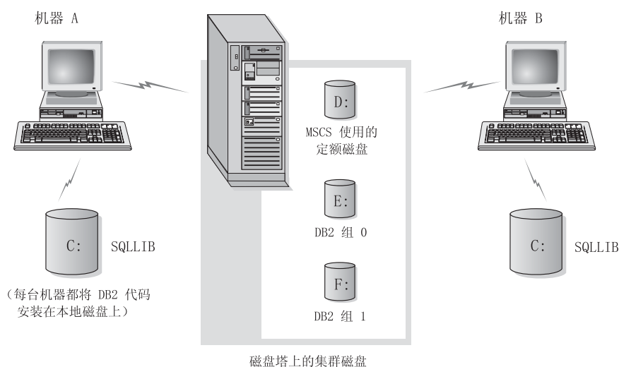
图 3. 示例 MSCS 配置
