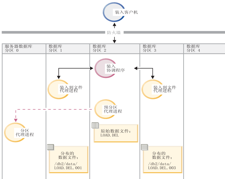
图 15. . 此图说明发出以上命令后产生的行为。将使用数据库分区 0 上运行的 1 个分区代理程序将数据装入到数据库分区 1 和 3 中。
