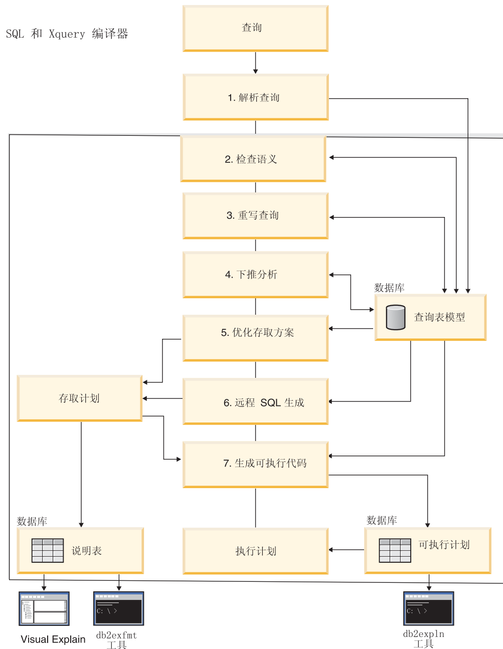
图 22. SQL 和 XQuery 编译器执行的步骤
