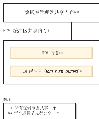
图 13. 使用多个逻辑节点时的 FCM 缓冲池
