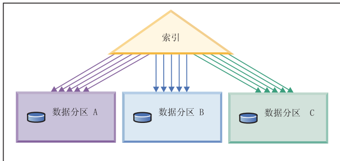
集群与分区键不匹配（以本地方式集群）
