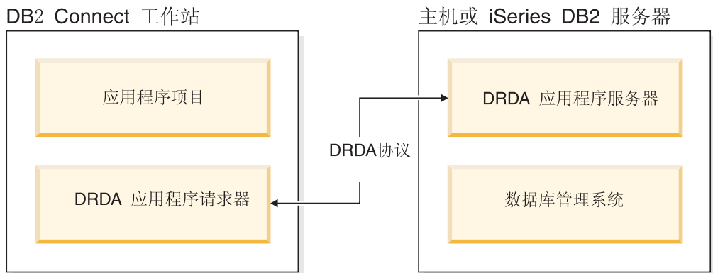
图 1. DB2 Connect 服务器与主机或 System i 服务器之间的数据流动
