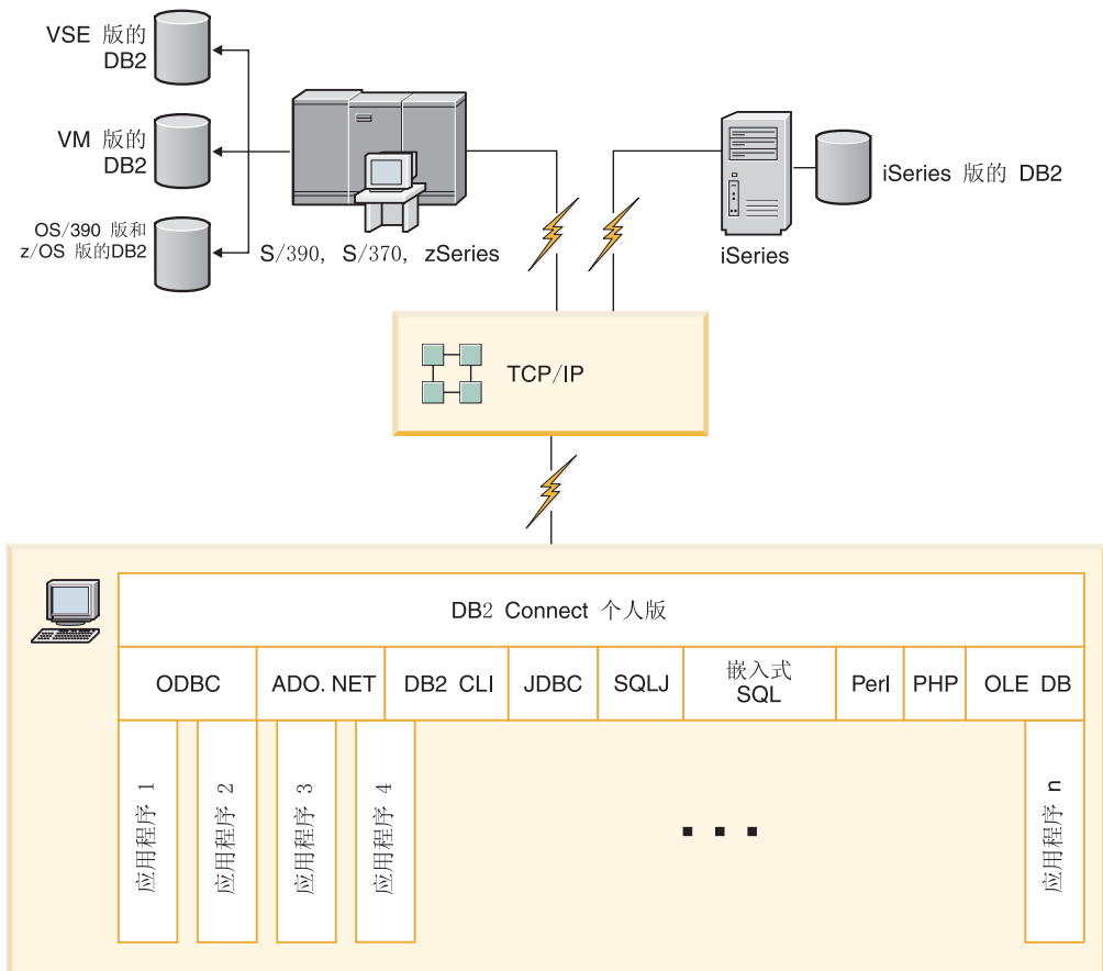
图 3. DB2 Connect 与主机或 System i 数据库服务器之间的直接连接。
