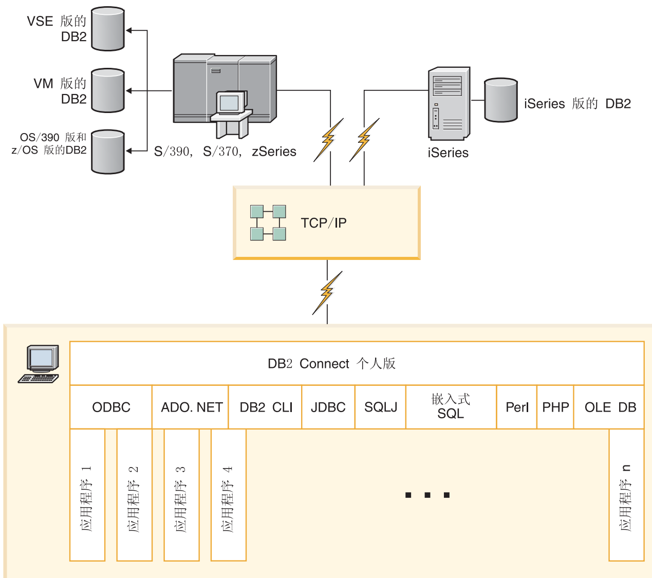
图 4. DB2 Connect 与主机或 System i 数据库服务器之间的直接连接
