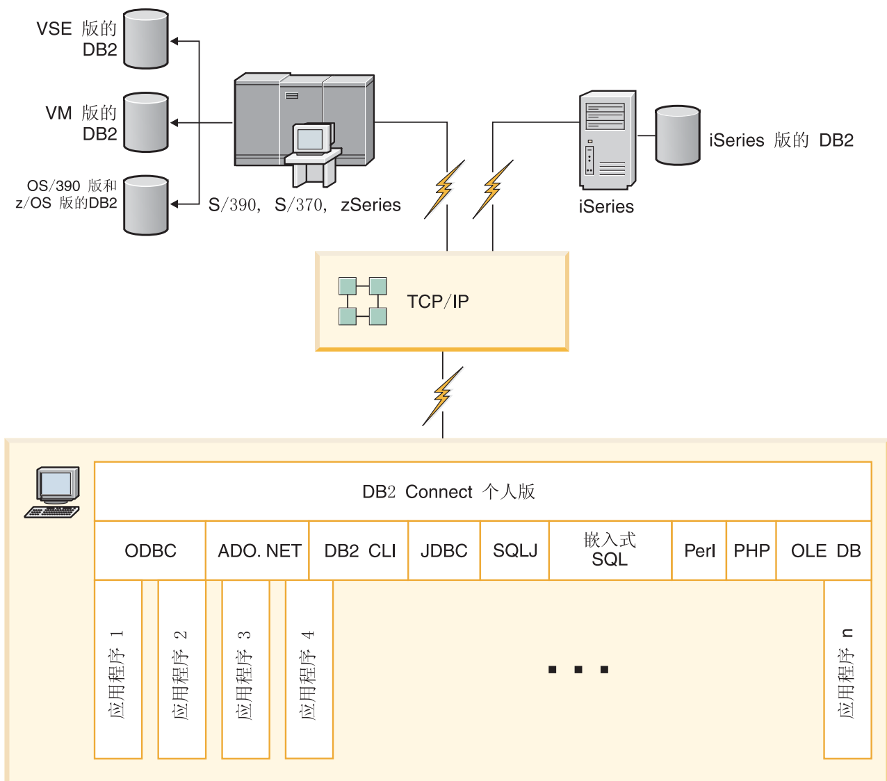
图 4. DB2 Connect 与主机或 System i 数据库服务器之间的直接连接
