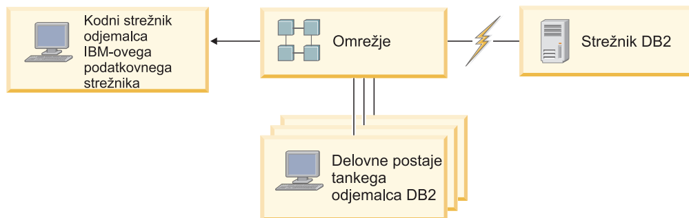
Slika 1. Značilna topologija tankega odjemalca, ki uporablja odjemalca IBM Data Server Client
