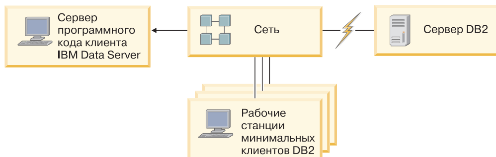
Рисунок 1. Типичная топология минимального клиента при использовании клиента IBM Data Server
