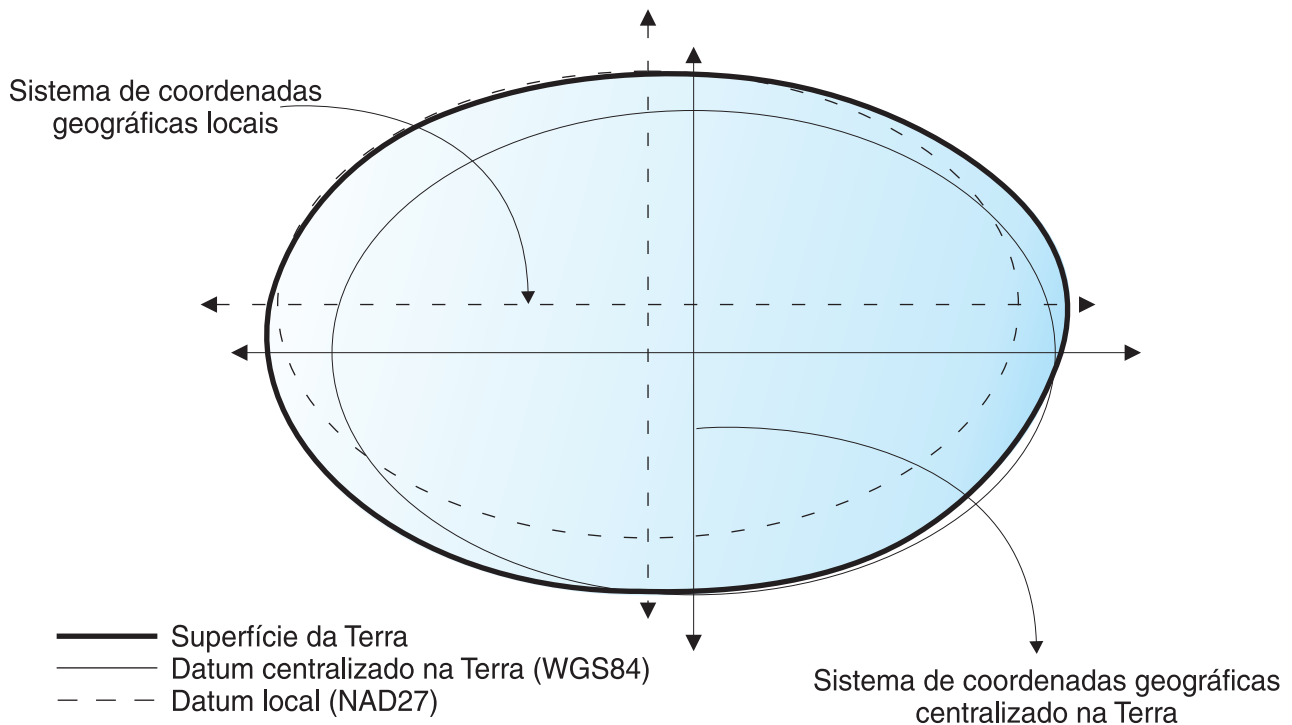
Figura 11. Alinhamentos de datums
