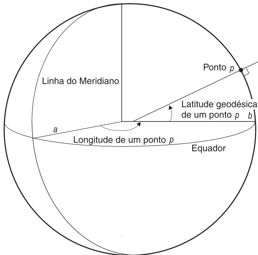
Figura 17. Ângulos de latitude e longitude geodésicas
