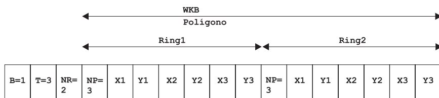
Figura 58. Representação geométrica em formato NDR. (B=1) do polígono tipo (T=3) com 2 lineares (NR=2), em que cada anel possui 3 pontos (NP=3).
