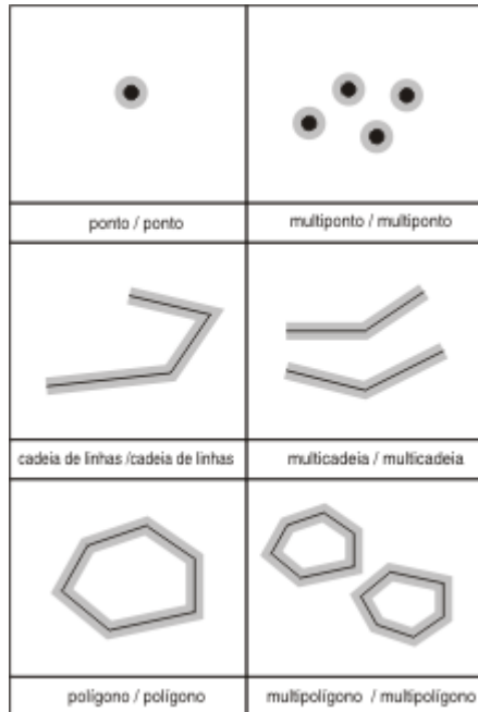
Figura 49. ST_Equals. As geometrias escuras representam a geometria a; as geometrias cinzas representam a geometria b. Em todos os casos, a geometria a é igual à geometria b.
