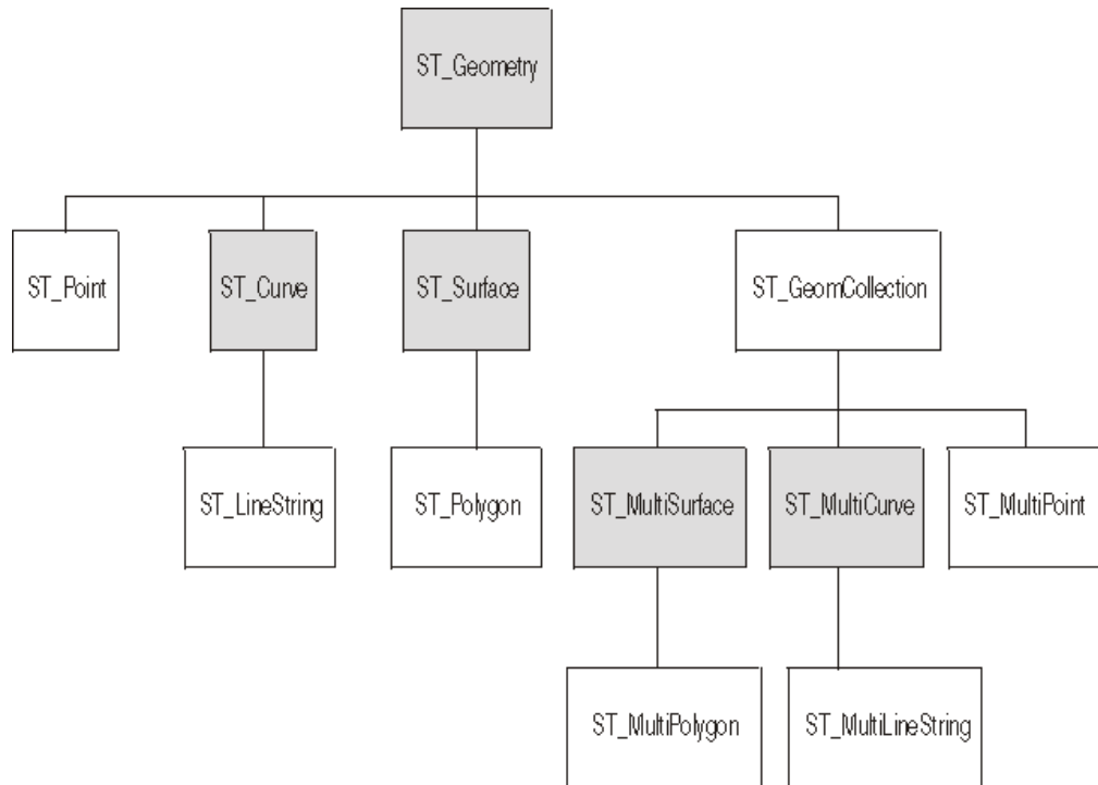
Figura 12. Hierarquia dos tipos de dados espaciais. Tipos de dados em caixas brancas podem ser instanciados. Os tipos de dados nomeados nas caixas sombreadas não são instanciáveis.
