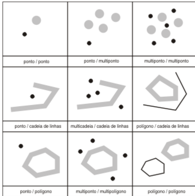
Figura 50. ST_Disjoint. As geometrias escuras representam a geometria a; as geometrias cinzas representam a geometria b. Em todos os casos, a geometria a e a geometria b são desconectadas uma da outra.
