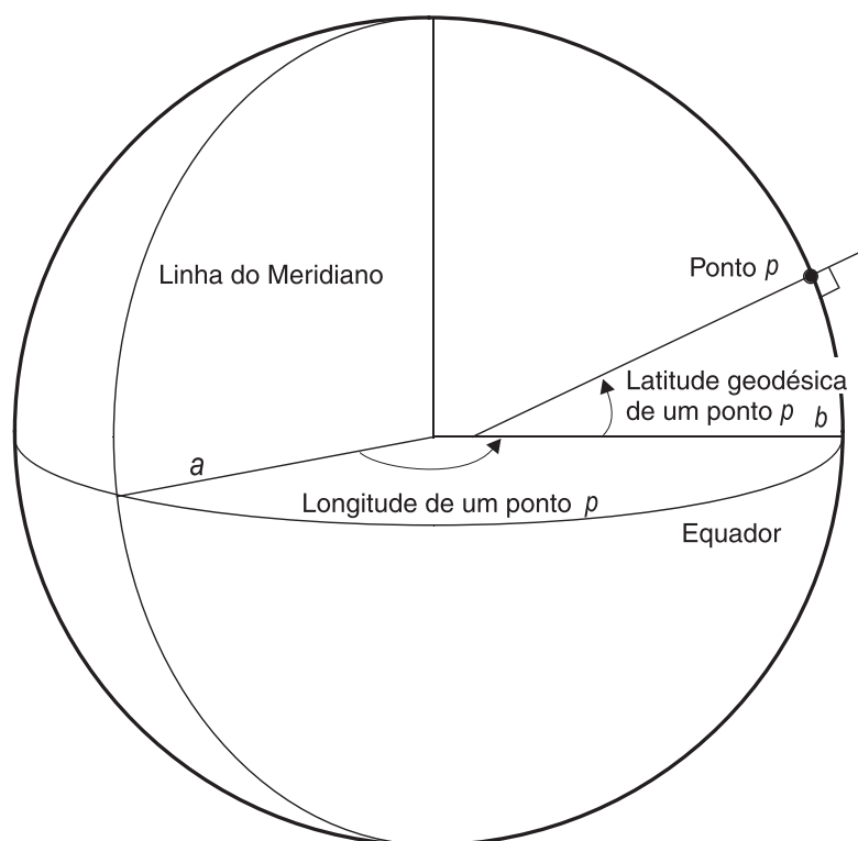
Figura 17. Ângulos de latitude e longitude geodésicas
