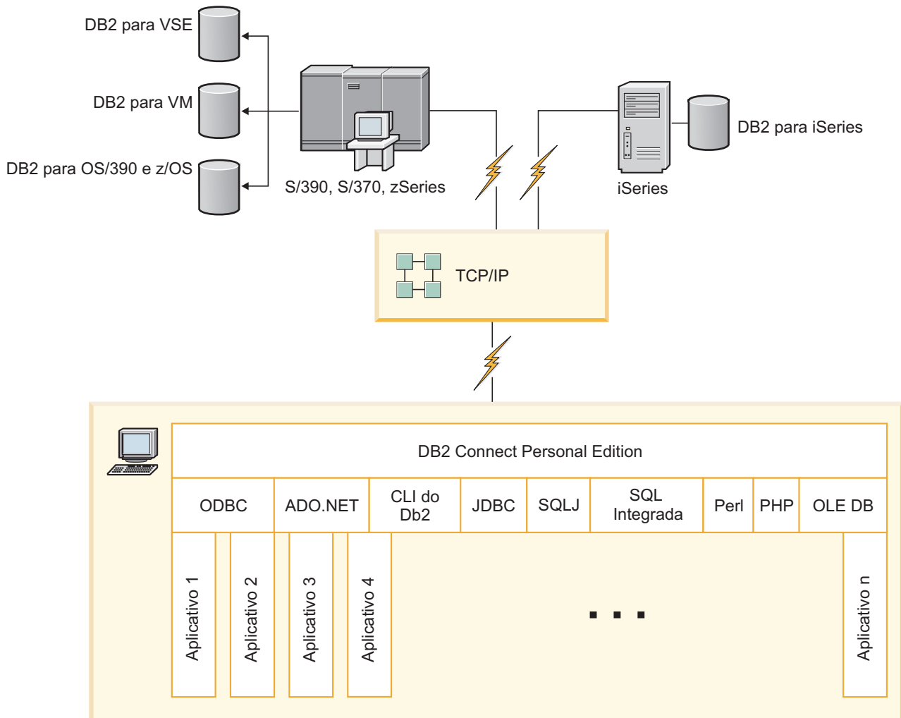
Figura 4. Conexão Direta entre o DB2 Connect e um Servidor de Banco de Dados do Host ou do System i
