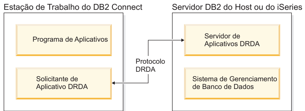
Figura 1. Fluxo de Dados entre um Servidor DB2 Connect e um Servidor Host ou System i
