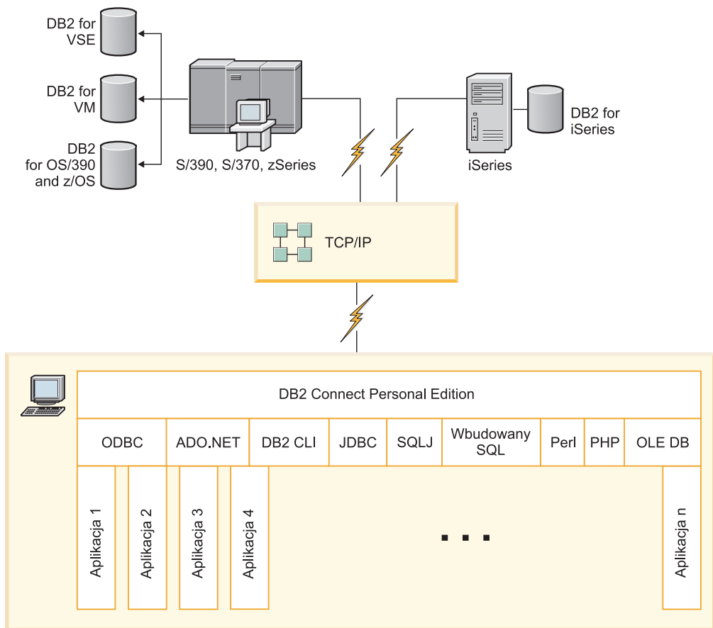
Rysunek 3. Bezpośrednie połączenie między programem DB2 Connect a serwerem bazy danych hosta lub systemu System i
