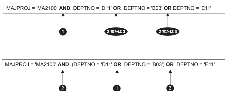
図 13. 検索条件の評価順序
