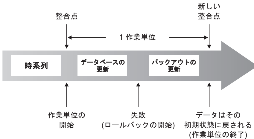
図 6. ROLLBACK ステートメントの作業単位
