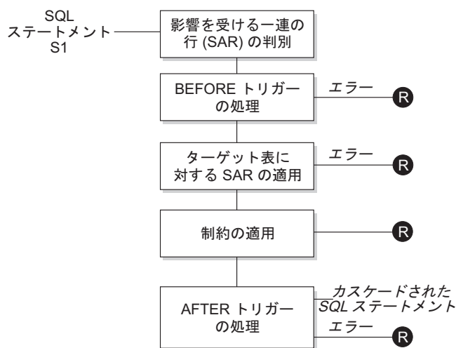
図 19. 関連するトリガーと制約を伴うステートメントの処理
