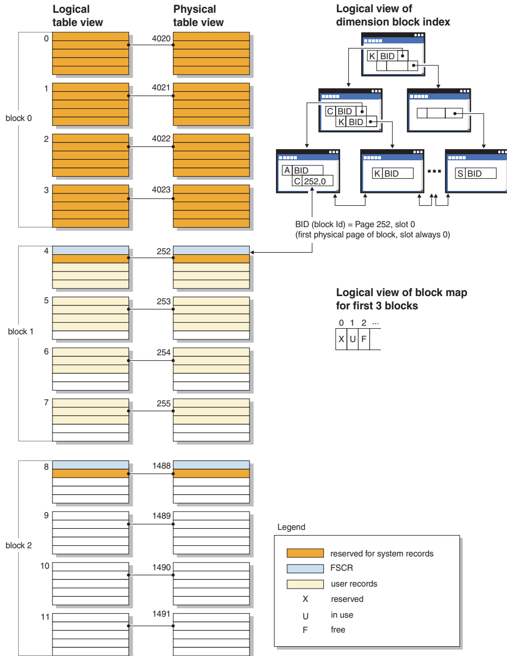
図 53. MDC 表の論理表、レコード、および索引構造
