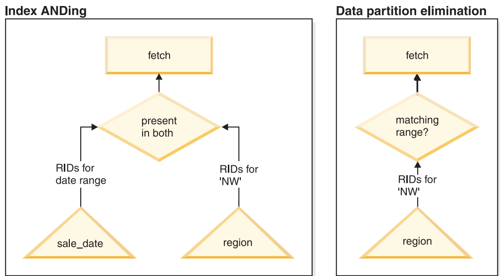
図 49. 表のパーティション化と索引 AND 演算の両方のオプティマイザーの決定パス
