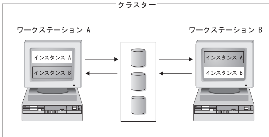
図 5. 相互テークオーバー構成
