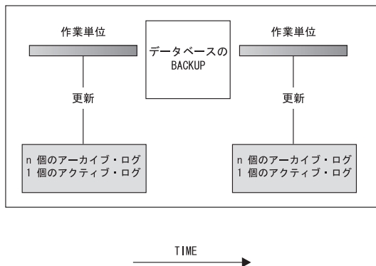
図2. ロールフォワード・リカバリーでのアクティブ・ログおよびアーカイブ・データベース・ログ：長時間実行しているトランザクションの場合には、複数のアクティブ・ログが生じる可能性があります。
