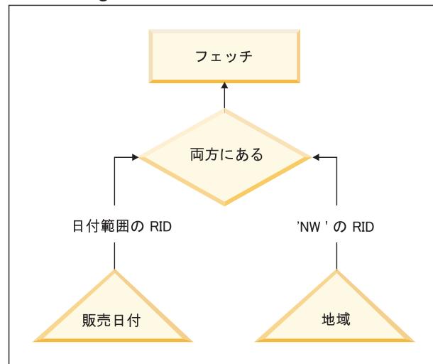
図 30. 表のパーティション化と索引 AND 演算の両方の最適化の決定パス
