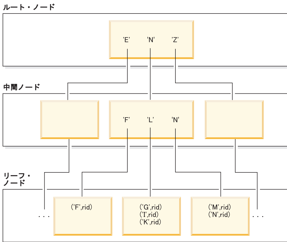
図 7. B+ ツリー構造
