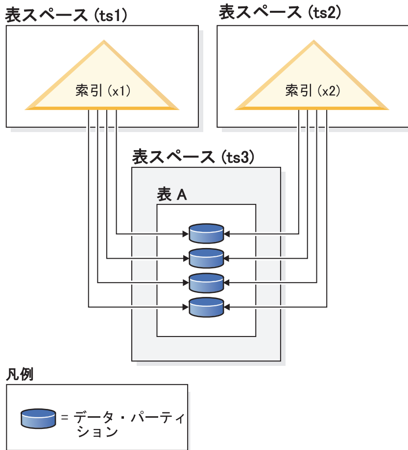
図 16. パーティション表上の索引の動作
