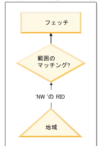
図 30. 表のパーティション化と索引 AND 演算の両方の最適化の決定パス
