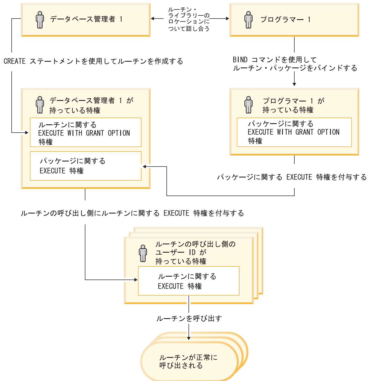
図3. ルーチンに関する EXECUTE 特権の管理
