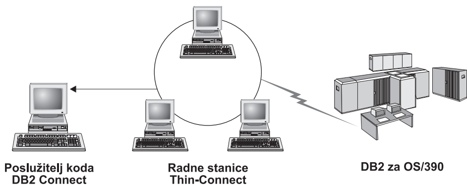
Slika 2. Tipična topologija tankog klijenta koji koristi DB2 Connect Personal Edition
