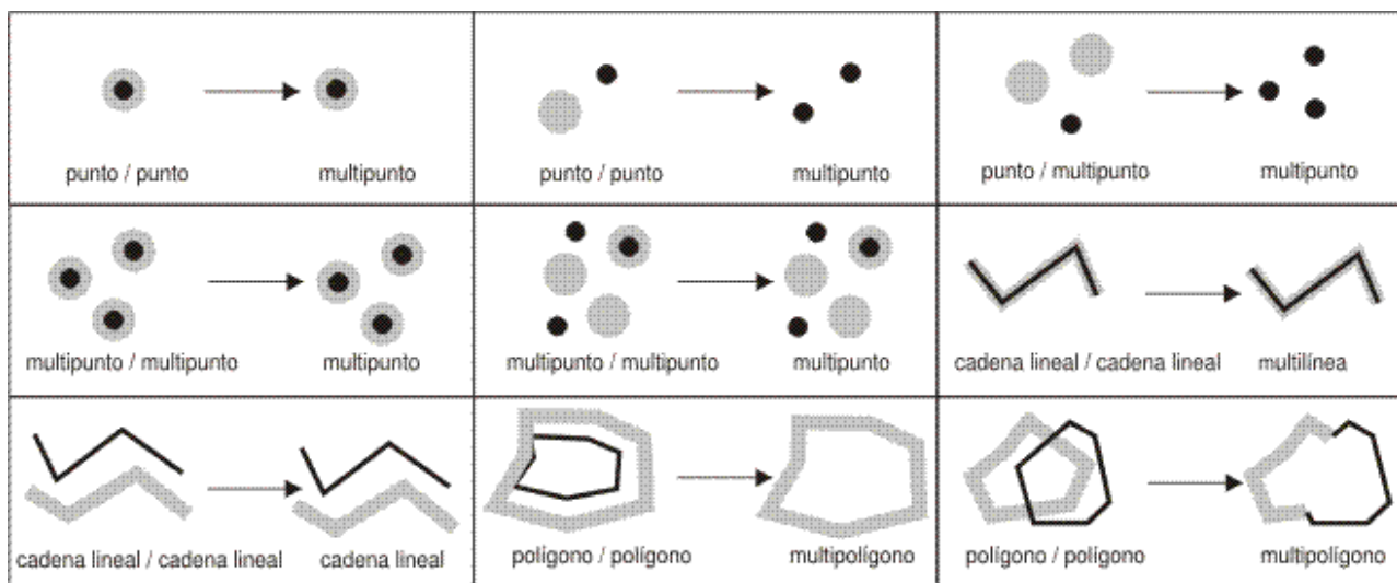
Figura 55. ST_Union
