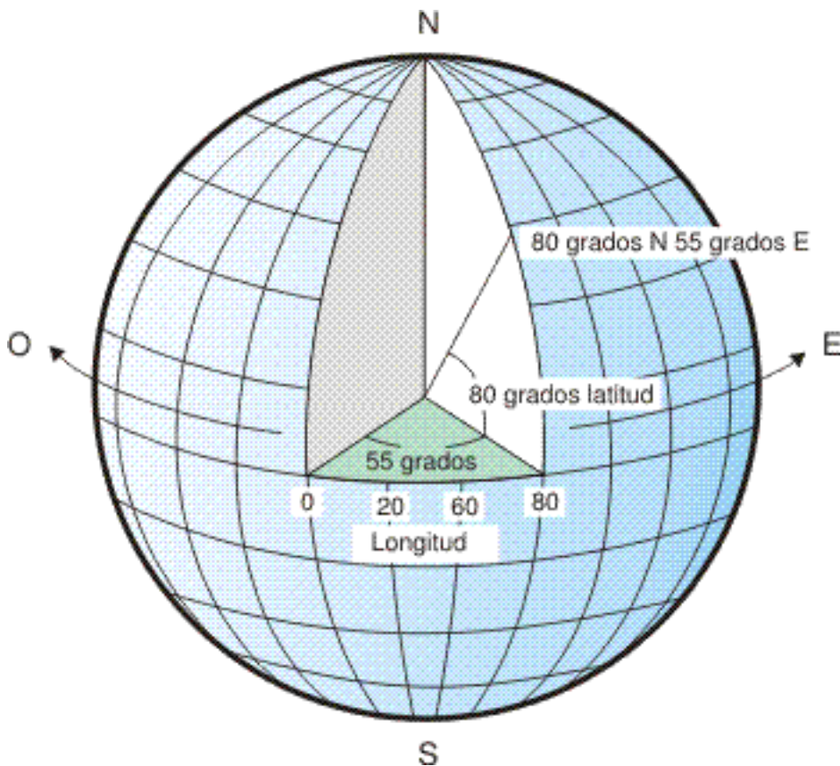
Figura 6. Un sistema de coordenadas geográficas
