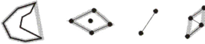
Figura 52. ST_ConvexHull
