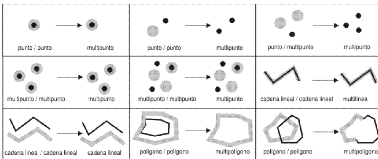
Figura 55. ST_Union
