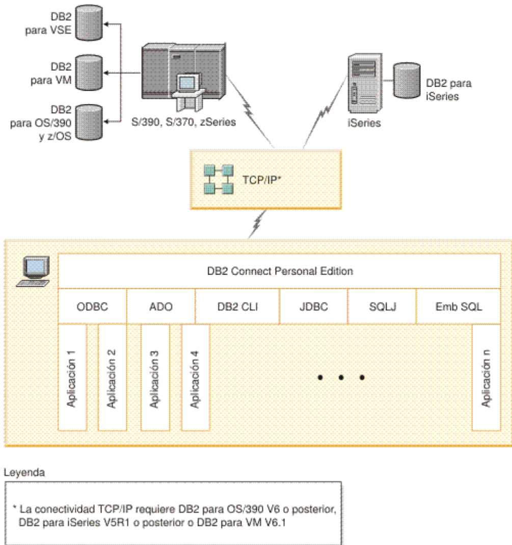
Figura 3. Conexión directa entre DB2 Connect y un servidor de bases de datos de sistema principal o System i
