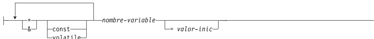
Figura 1. Diagrama de sintaxis
