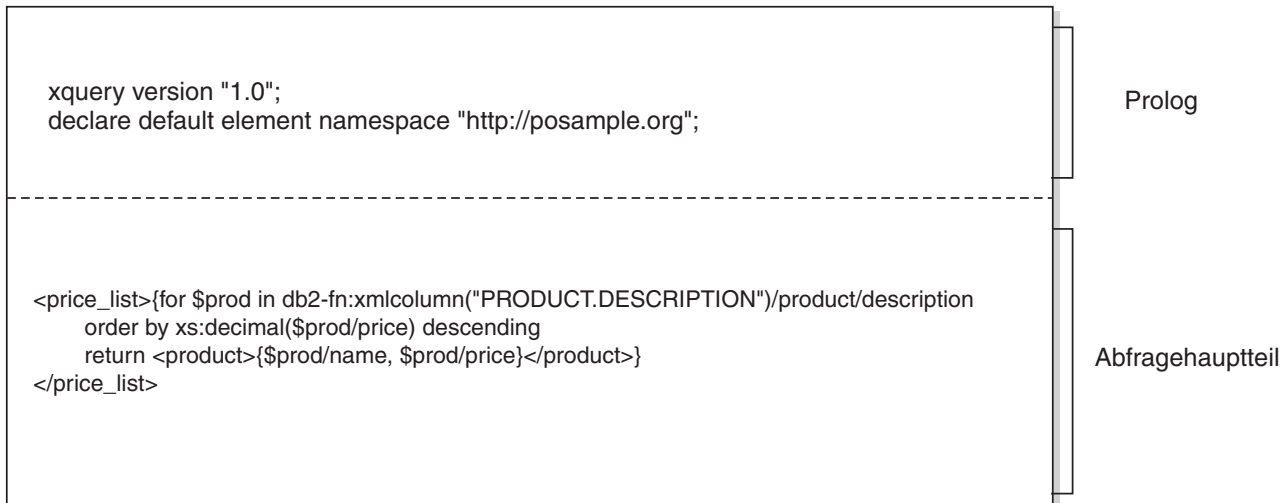
Abbildung 1. Struktur einer typischen XQuery-Abfrage
