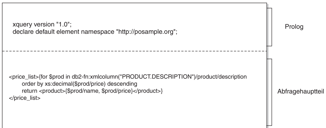
Abbildung 4. Struktur einer typischen XQuery-Abfrage
