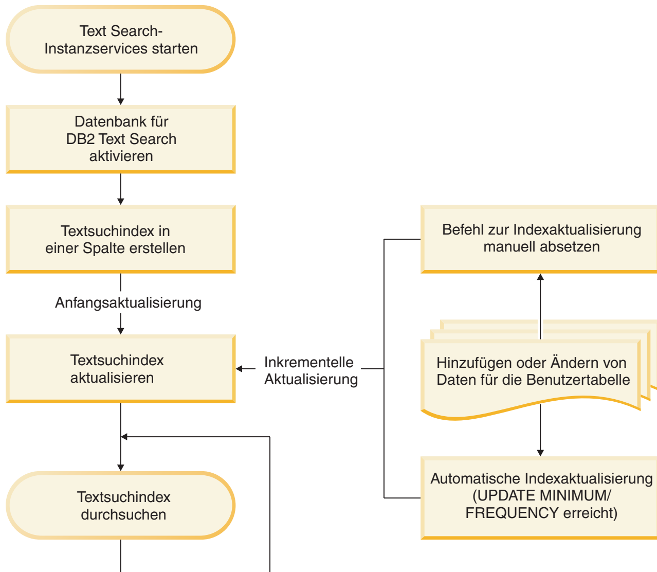
Abbildung 2. Einrichten von Textsuchindizes zum Durchsuchen
