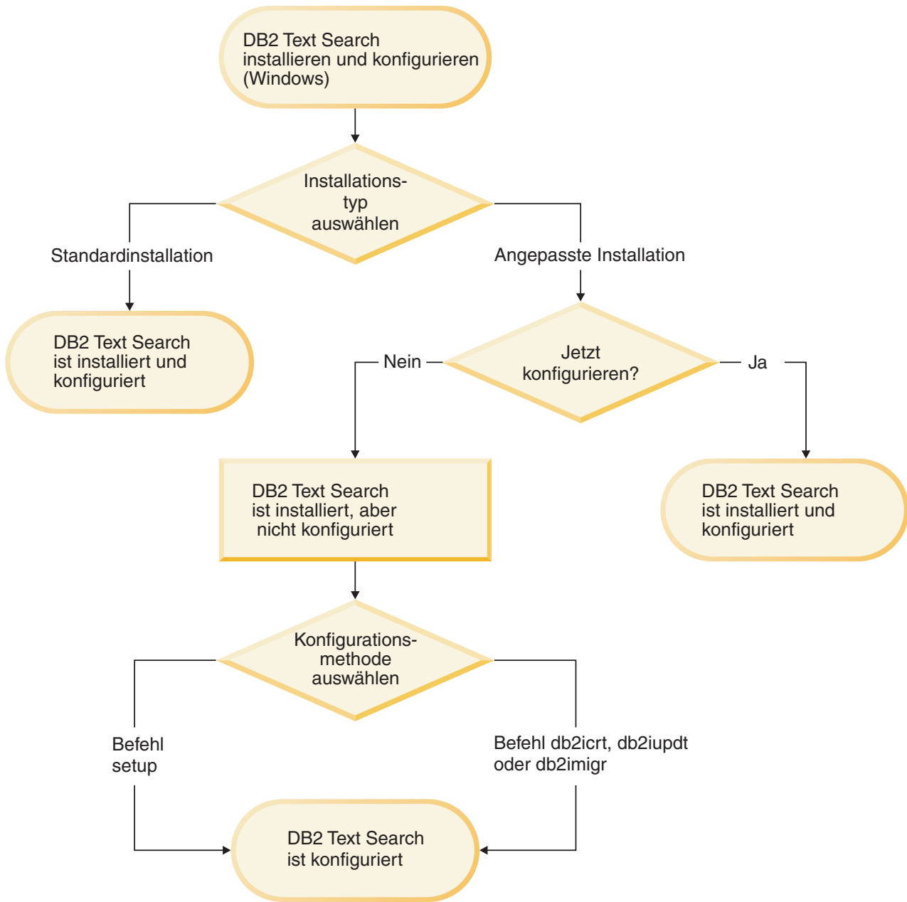
Abbildung 4. Installation und Konfiguration auf Windows-Plattformen
