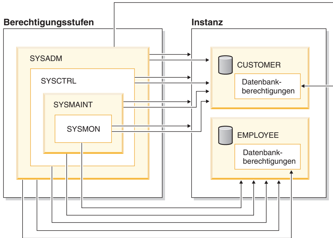
Abbildung 1. Hierarchie der Berechtigungen
