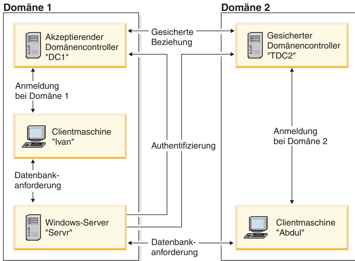
Abbildung 5. Authentifizierung in Windows-Domänen
