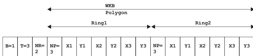
Abbildung 58. Geometriedarstellung im NDR-Format. (B=1) des Typs "Polygon" (T=3) mit 2 Linearen (NR=2), wobei jeder Ring drei Punkte hat (NP=3).
