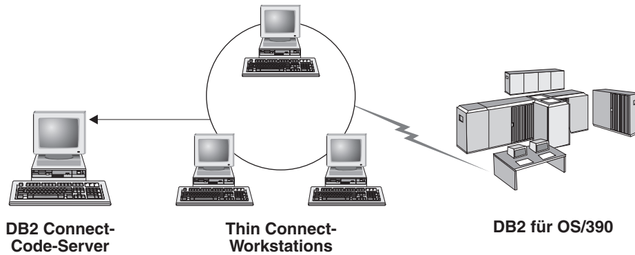
Abbildung 2. Eine typische Thin Client-Topologie unter Verwendung von DB2 Connect Personal Edition
