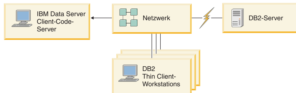
Abbildung 1. Eine typische Thin Client-Topologie unter Verwendung von IBM Data Server Client
