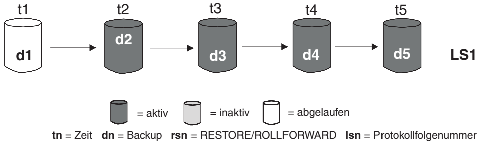
Abbildung 14. Abgelaufene Datenbankbackups
