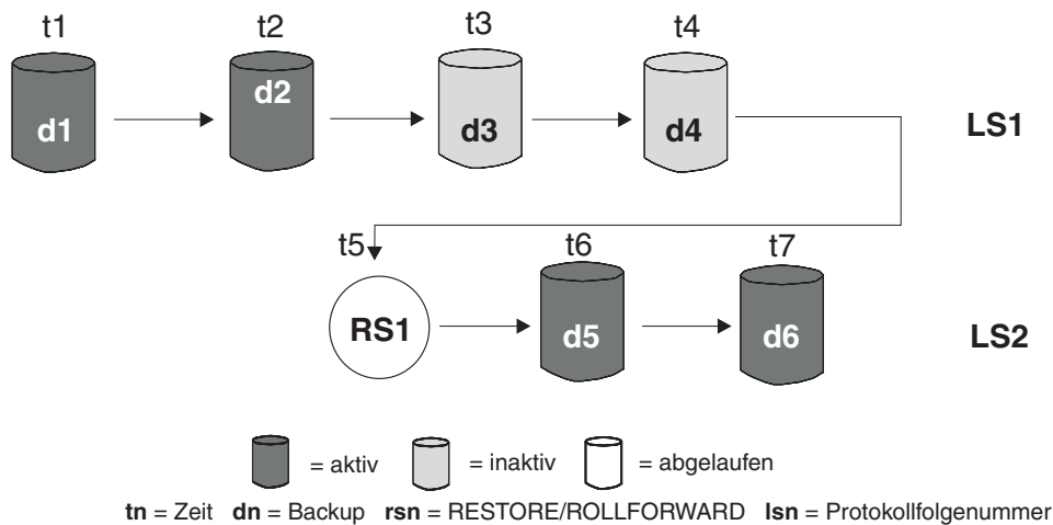
Abbildung 13. Inaktive Datenbankbackups
