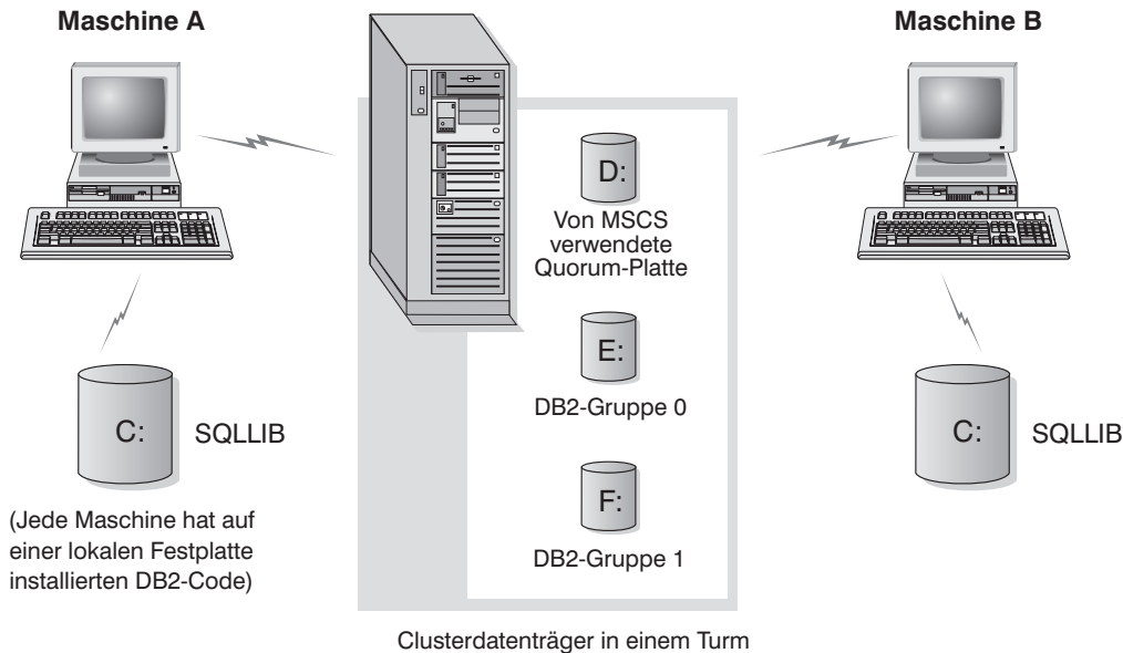
Abbildung 3. Beispiel für eine MSCS-Konfiguration
