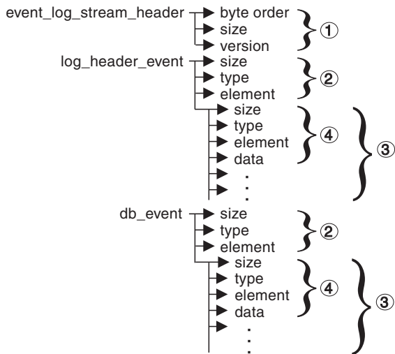
Abbildung 2. Datenstrom eines Ereignismonitors
