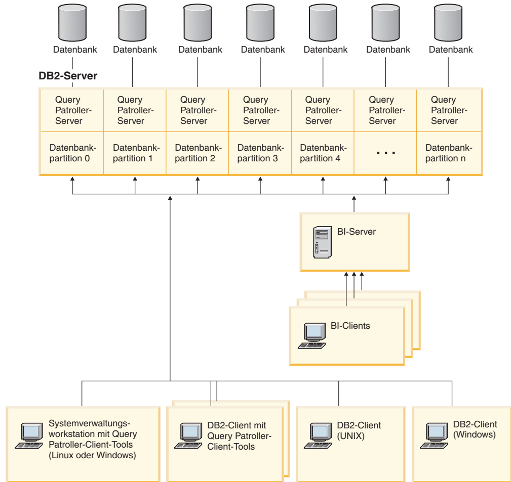
Abbildung 3. Partitionierte Query Patroller-Datenbankinstallationsumgebung
