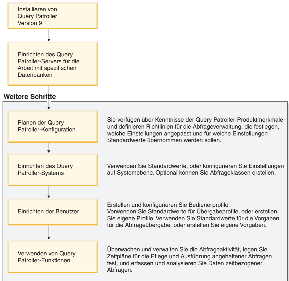
Abbildung 4. Übersicht über die Query Patroller-Verwaltungstasks
