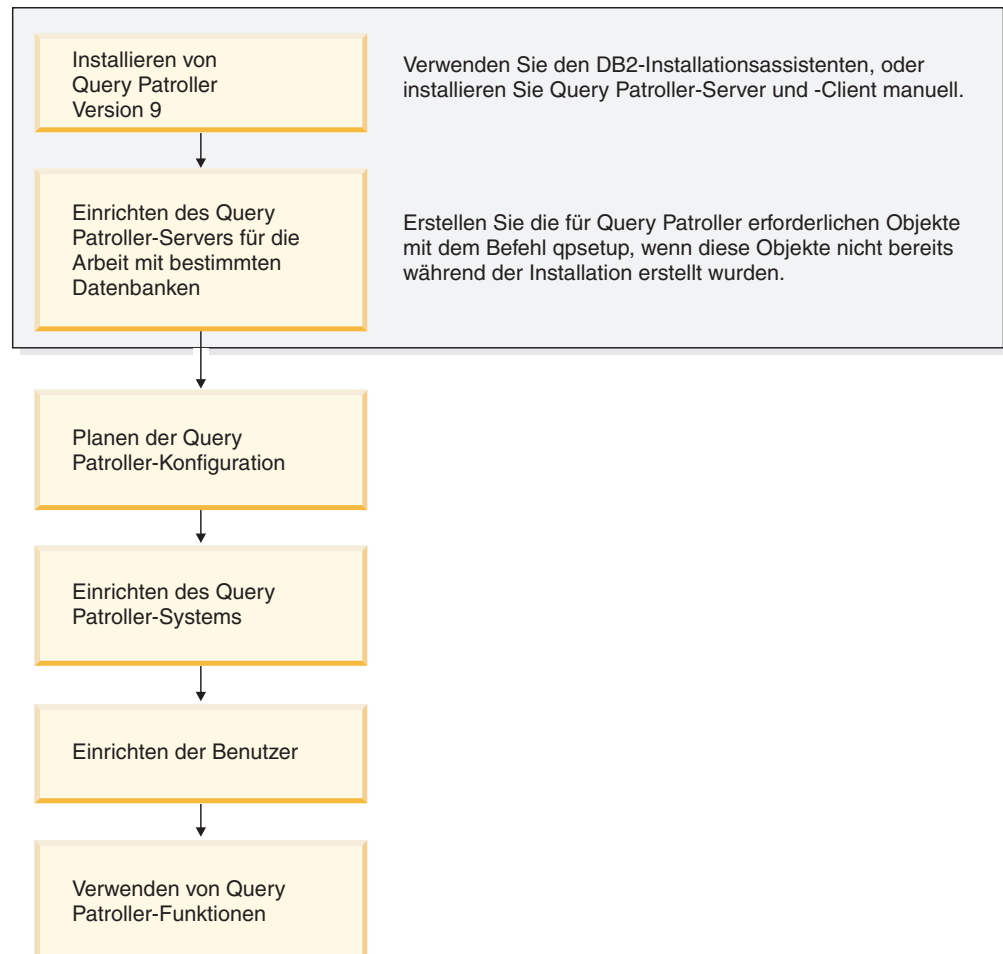
Abbildung 1. Übersicht über die Query Patroller-Installationstasks
