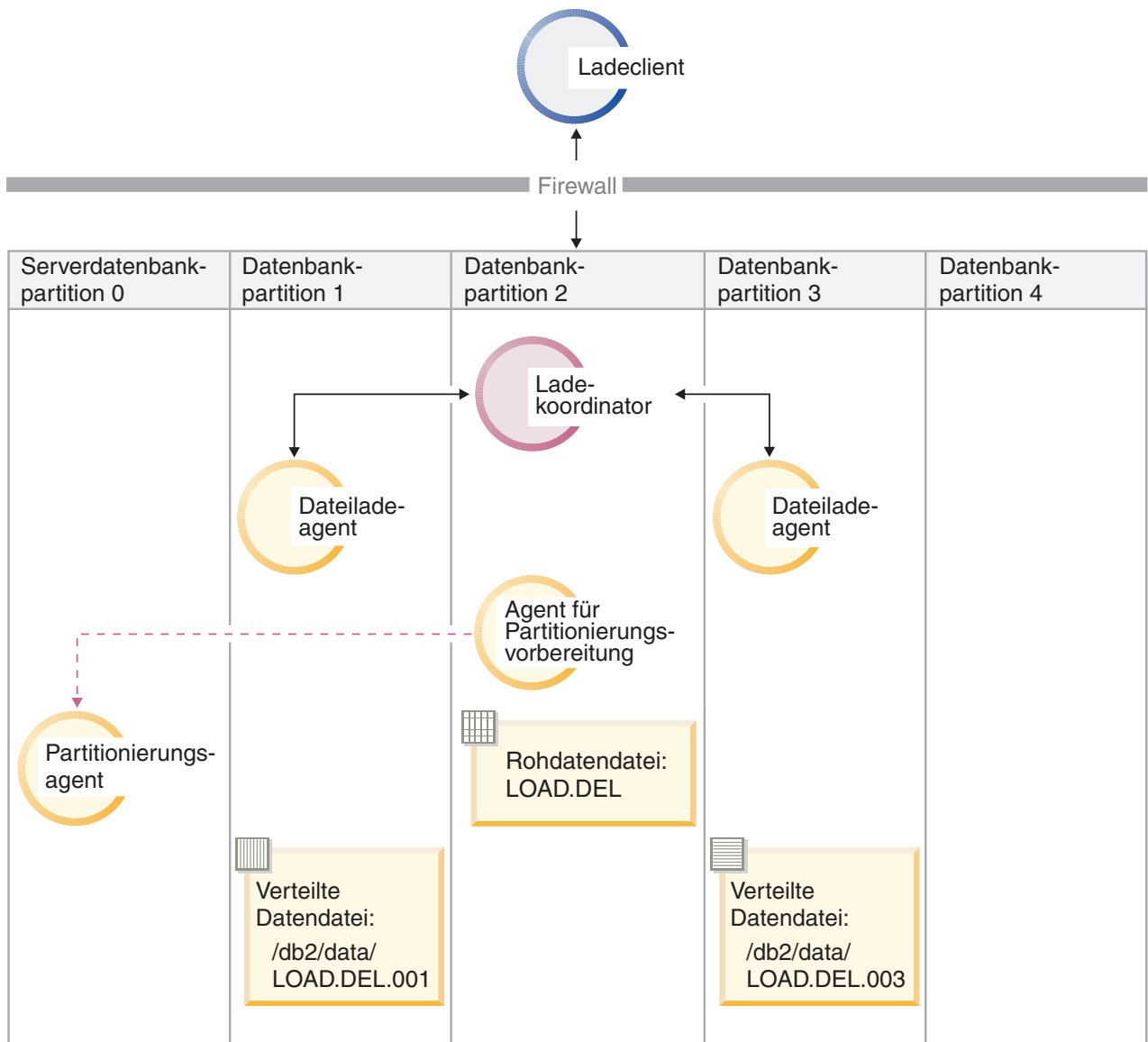
Abbildung 15. Diese Abbildung veranschaulicht das Verhalten, das sich bei Ausführung des vorstehenden Befehls ergibt. Die Daten werden auf die Datenbankpartitionen 1 und 3 geladen, wobei ein Partitionierungsagent verwendet wird, der auf Datenbankpartition 0 aktiv ist.
