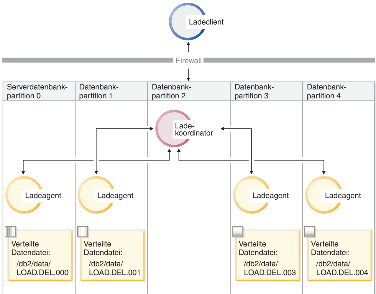
Abbildung 16. Diese Abbildung veranschaulicht das Verhalten, das sich bei Ausführung des vorstehenden Befehls ergibt. Die verteilten Daten werden auf alle Datenbankpartitionen geladen, auf denen TABLE1 definiert ist.
